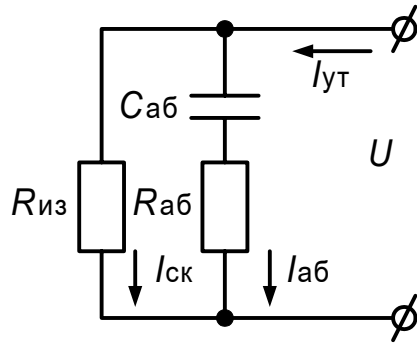
Рис. 5. Электрическая схема замещения диэлектрика: R_{из} – сопротивление изоляции; R_{аб} , C_{аб} – соответственно абсорбционные сопротивление и емкость; U – приложенное напряжение
