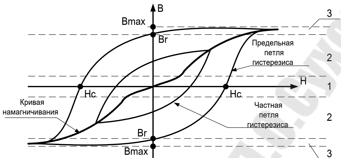
Рис. 16. Процессы намагничивания ферромагнетика
