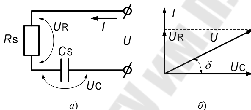
Рис. 9. Последовательная схема замещения диэлектрика (а) и векторная диаграмма последовательной схемы замещения (б)
