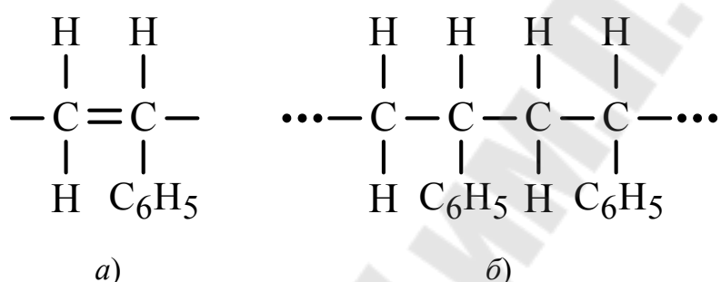
Рис. 11. Молекула стирола-мономера (а) и молекула полистирола (б)
