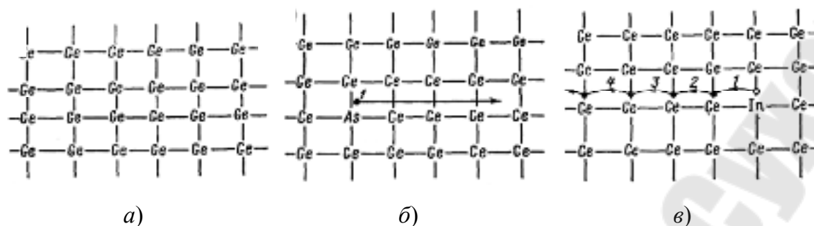
Рис. 13. Кристаллическая решетка германия: a – без примесей; б – с донорной примесью мышьяка; в – с акцепторной примесью индия (1–4 – номера электронов)
