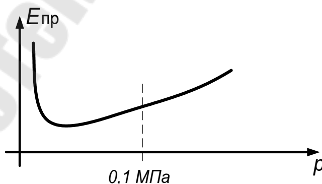
Рис. 10. Зависимость электрической прочности воздуха от давления
