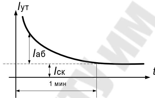
Рис. 6. Процесс изменения тока утечки диэлектрика при приложении напряжения
