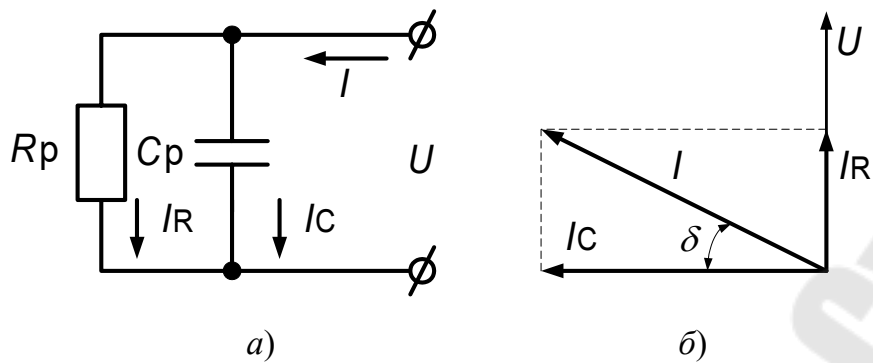
Рис. 8. Параллельная схема замещения диэлектрика (а) и векторная диаграмма параллельной схемы замещения (б)
