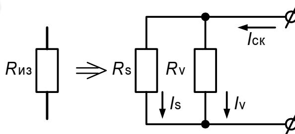
Рис. 7. Составляющие сопротивления изоляции диэлектрика
