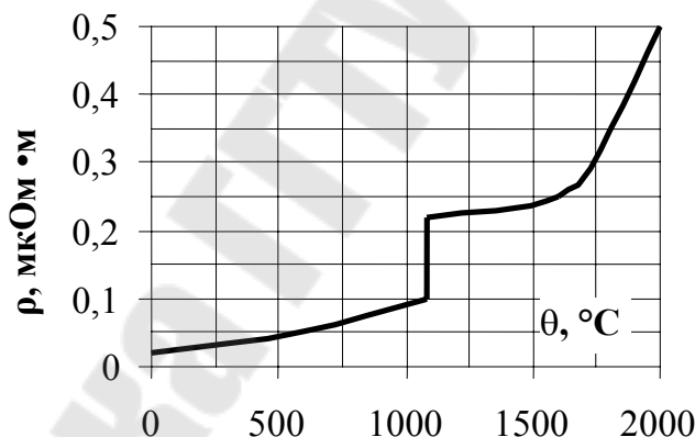
Рис. 12. Зависимость \rho = f(\theta) для меди
