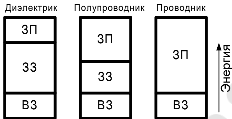
Рис. 3. Энергетические диаграммы диэлектрика: ЗП – зона проводимости; ЗЗ – запрещенная зона; ВЗ – валентная зона
