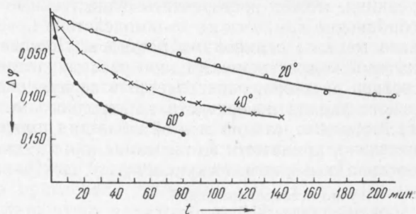
Рис. 3. Зависимость потенциала от времени при переходе с верхней ветви кривой перенапряжения на нижнюю в растворе 1 н \text{H}_2\text{SO}_4 при разных температурах
