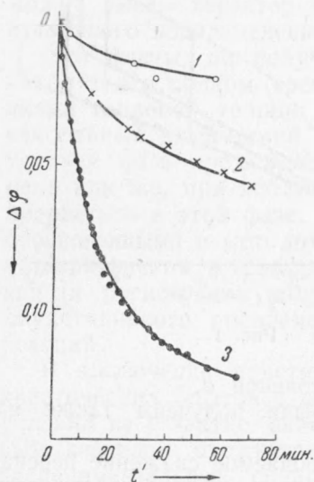
Рис. 2. Зависимость потенциала от времени при переходе с верхней ветви кривой перенапряжения на нижнюю в растворах: 1—1 н \text{H}_2\text{SO}_4 ; 2—1 н \text{HCl} ; 3—1 н \text{H}_2\text{SO}_4 + 0,1 н \text{KJ}
