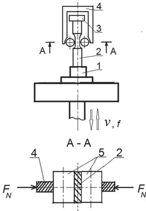
Рисунок 4 — Схема испытаний на КМУ на вибростенде: 1 — захват; 2 — образец; 3 — груз; 4 — динамометрическая скоба; 5 — контрообразцы-ролики
