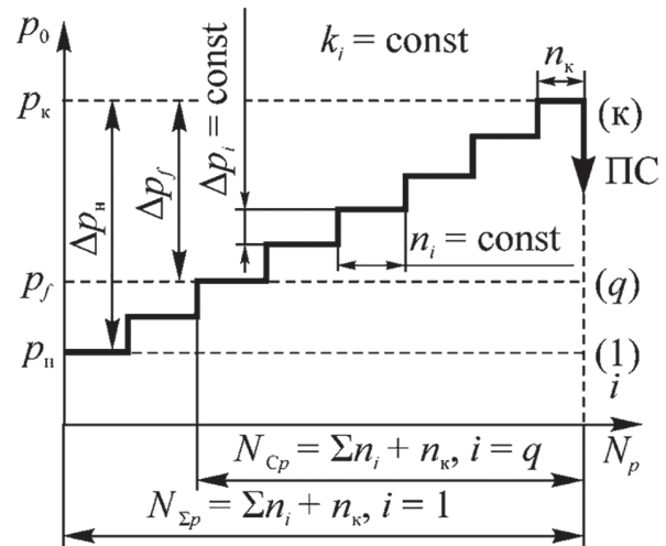
Рисунок 2 — Программа ступенчатого нагружения и основные характеристики сопротивления контактной усталости Figure 2 — Step loading program and main characteristics of contact fatigue resistance
