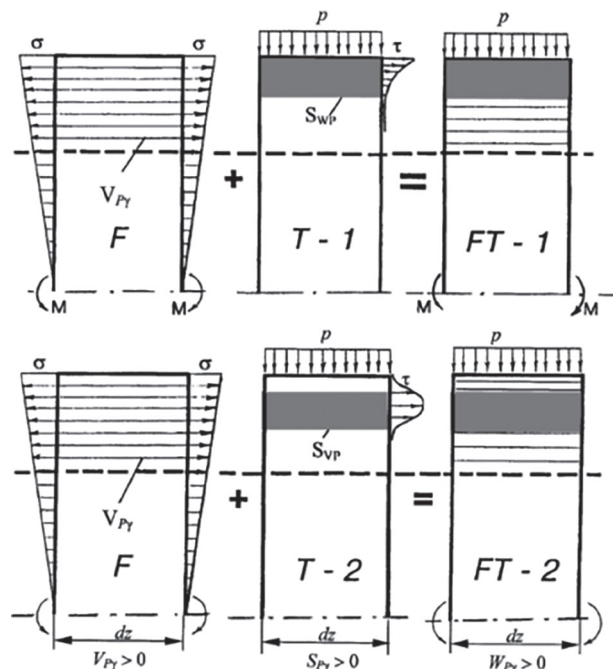
Рисунок 1 — Схемы формирования опасных объемов при испытаниях на трение ( S_{P\gamma} > 0 ), механическую усталость ( V_{P\gamma} > 0 ) и при износоусталостных испытаниях ( W_{P\gamma} > 0 ) Figure 1 — Formation schemes of dangerous volumes during friction tests ( S_{P\gamma} > 0 ), mechanical fatigue ( V_{P\gamma} > 0 ) and wear and fatigue tests ( W_{P\gamma} > 0 )
