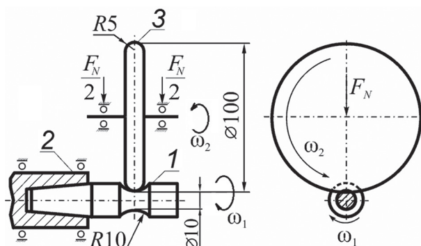
Рисунок 3 — Схема испытаний на контактную усталость: 1 — образец; 2 — шпиндель; 3 — контробразец (ролик с профильным радиусом) Figure 3 — Rolling fatigue test scheme: 1 — sample; 2 — spindle; 3 — control sample (roller with profile radius)
