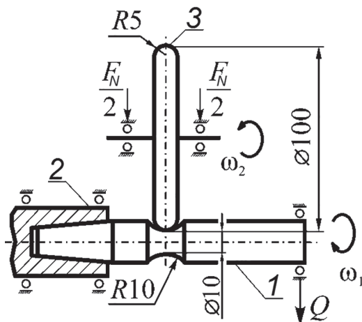
Рисунок 5 — Схема испытаний на КМУ: 1 — образец; 2 — шпиндель; 3 — контрообразец (ролик с профильным радиусом) Figure 5 — MRF test scheme: 1 — sample; 2 — spindle; 3 — control sample (roller with profile radius)
