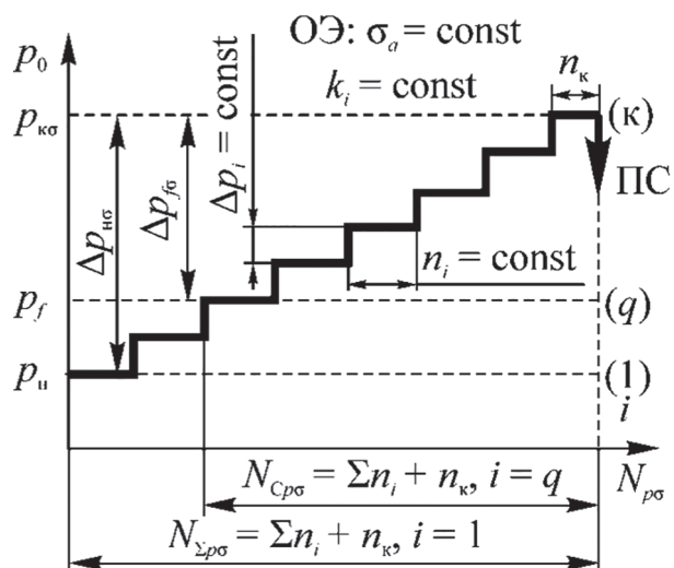
Рисунок 6 — Программа ступенчатого нагружения при КМУ и основные характеристики сопротивления КМУ:
