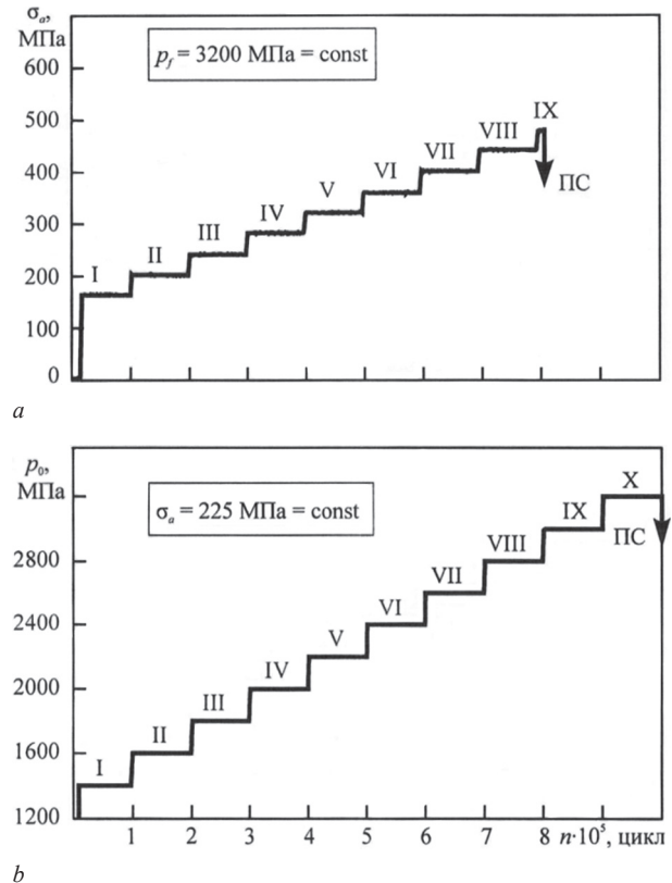
Рисунок 7 — Результаты испытаний на КМУ методом многоступенчатого нагружения при ПЭ (а) и при ОЭ (б) Figure 7 — Results of MRF tests by multi-stage loading at direct effect (a) and at back effect (b)
