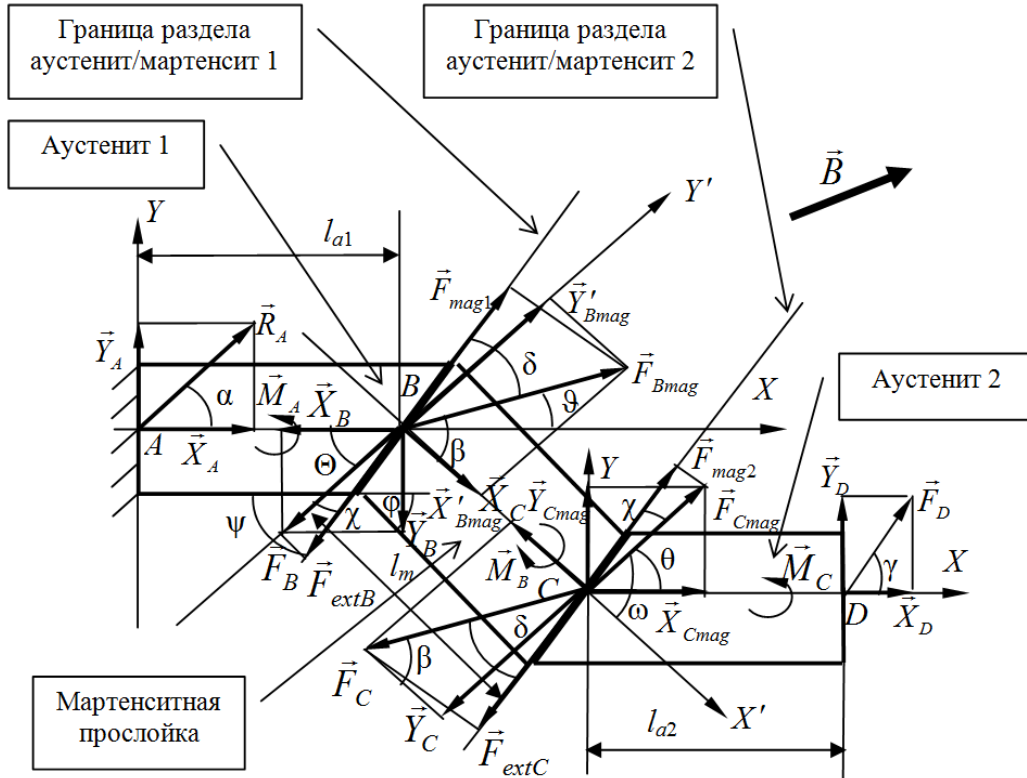
Рисунок 1.1 – Ферромагнитный призматический монокристаллический образец с эффектом памяти формы с мартенситной прослойкой, находящийся в жесткой заделке в магнитном поле
