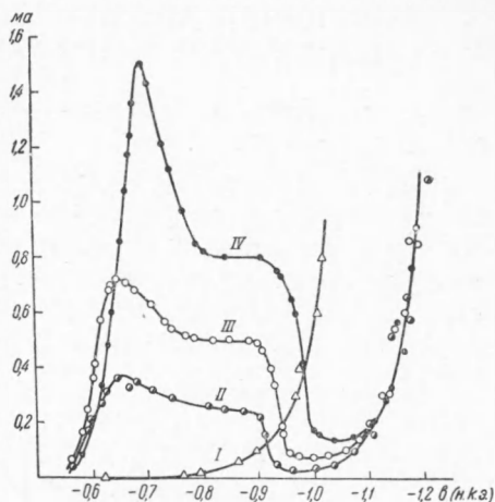
Рис. 4. Зависимость скорости восстановления хромовой кислоты от потенциала электрода в присутствии различных количеств серной кислоты. I — без добавки \text{H}_2\text{SO}_4 , II — 2,5 г/л \text{H}_2\text{SO}_4 , III — 5 г/л \text{H}_2\text{SO}_4 , IV — 10 г/л \text{H}_2\text{SO}_4
