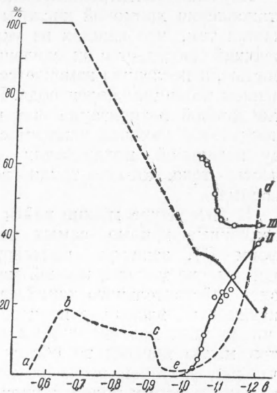
Рис. 3. Распределение тока в процессе электролиза между реакциями: I — \text{CrO}_4^{2-} + 8\text{H}^+ + 3\text{e} \rightarrow \text{Cr}^{3+} + 4\text{H}_2\text{O} ; II — \text{CrO}_4^{2-} + 8\text{H}^+ + 6\text{e} \rightarrow \text{Cr} + 4\text{H}_2\text{O} ; III — 2\text{H}^+ \rightarrow \text{H}_2 . Пунктир — кривая II рис. 4
