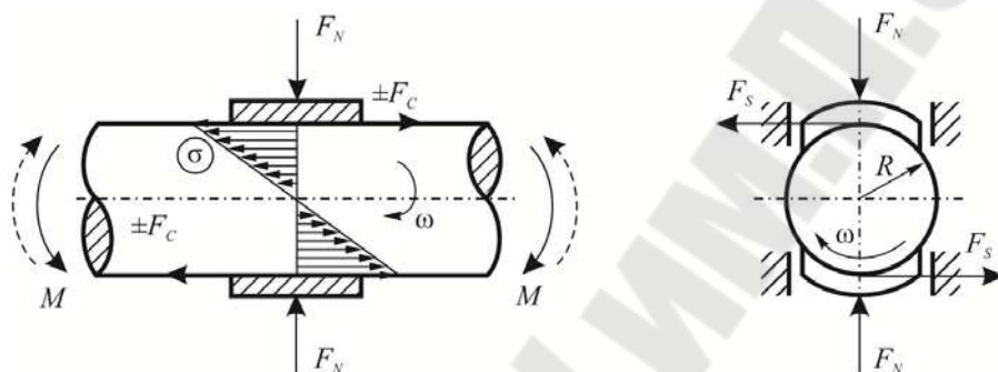
Рисунок 3.1а – Принципиальные схемы типичных трибофатических систем «твердое тело – твердое тело». Фрикционно-механическая усталость (ФМУ)
