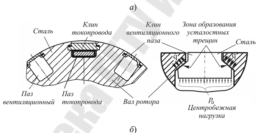
Рисунок 1.2 – Общий вид турбины (а) и схема вала ротора в зоне стыка пазовых клиньев (б)
