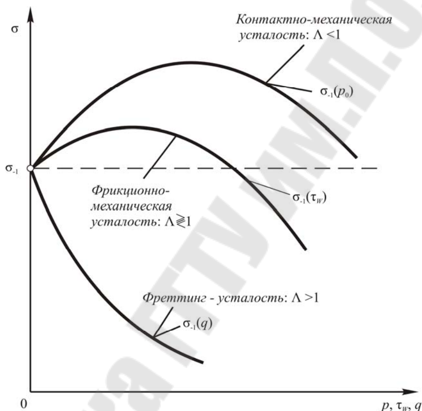
Рисунок 10.9 – Схема, поясняющая основные особенности \Lambda -взаимодействий при прямом эффекте (Л. А. Сосновский)
