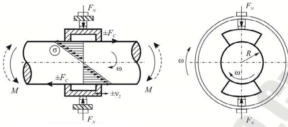
Рисунок 3.1в – Принципиальные схемы типичных трибофатических систем «твердое тело – твердое тело». Фреттинг-усталость (ФрУ)
