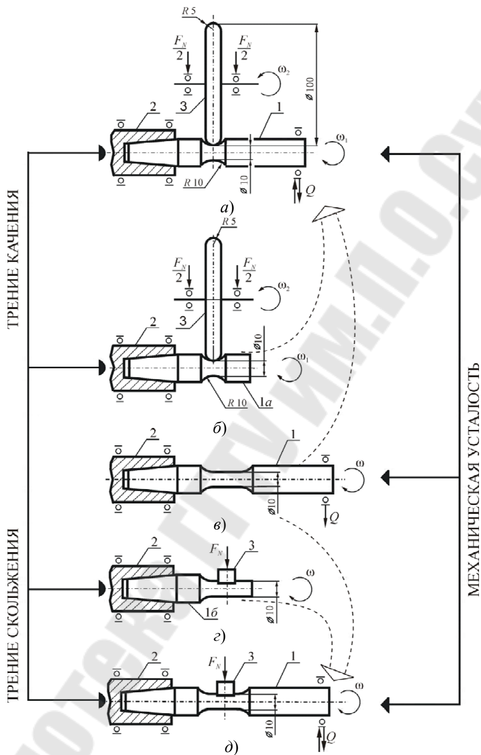
Рисунок 4.2 – Типичные схемы износоусталостных испытаний: 1, 1а, 1б – образец; 2 – шпиндель испытательной машины; 3 – контрообразец; Q – изгибающая нагрузка; F_N – контактная нагрузка; \omega_1 , \omega_2 – скорость вращения образца, контрообразца; а – контактно-механическая усталость; б – контактная усталость; в – механическая усталость; г – фрикционная усталость; д – фрикционно-механическая усталость
