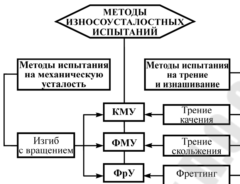
Рисунок 4.1 – Формирование методов износоусталостных испытаний при главном вращательном движении:
