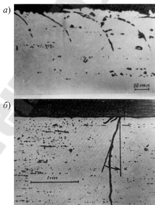
Рисунок 10.6 – Микротрещины в алюминиевом сплаве в первом периоде ( а ) (К. I. Nix, Т. С. Lindley); магистральная трещина во втором периоде ( б ) фреттинг-усталости (Р. R. Edwards)
