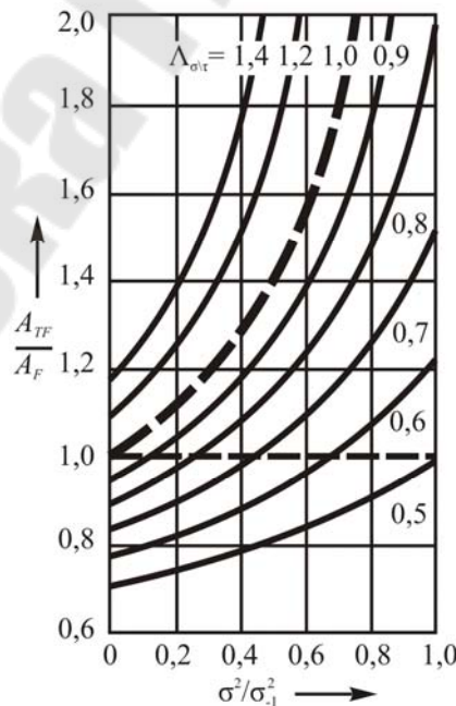
Рисунок 13.2 – К определению площади контакта
