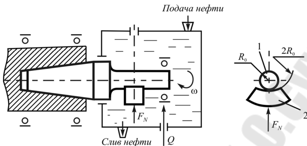
Рисунок 12.4 – Оригинальная модель системы «труба – поток жидкости под давлением»
