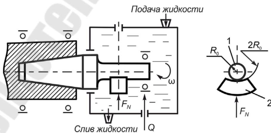
Рисунок 4.4 – Схема испытаний на коррозионно-эрозионную усталость
