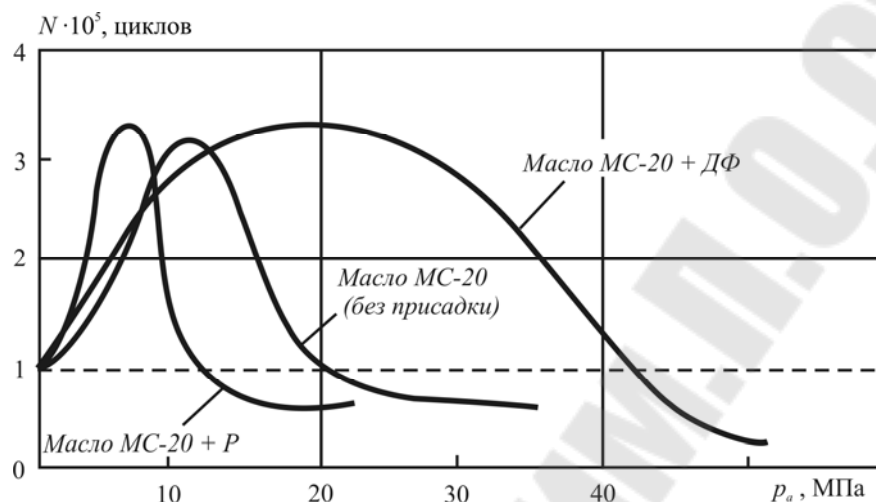
Рисунок 7.3 – Влияние давления при трении со смазочным материалом на долговечность образцов стали 45 при \sigma_a = 400 МПа ( \sim 1,25\sigma_{-1} ) (И. Г. Носовский и др.)
