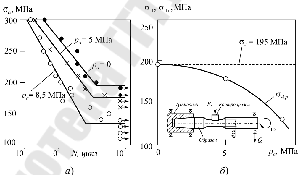
Рисунок 7.1 – Результаты износоусталостных испытаний системы «сталь 40Х – полиамид «Дуретан» ВКВ-30Н»:
