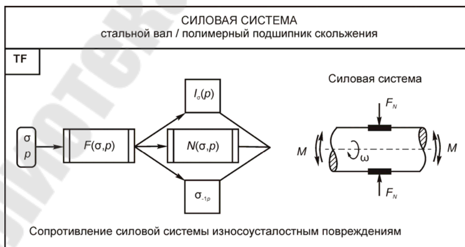
Рисунок 2.2 – К расчету трибофатической системы
