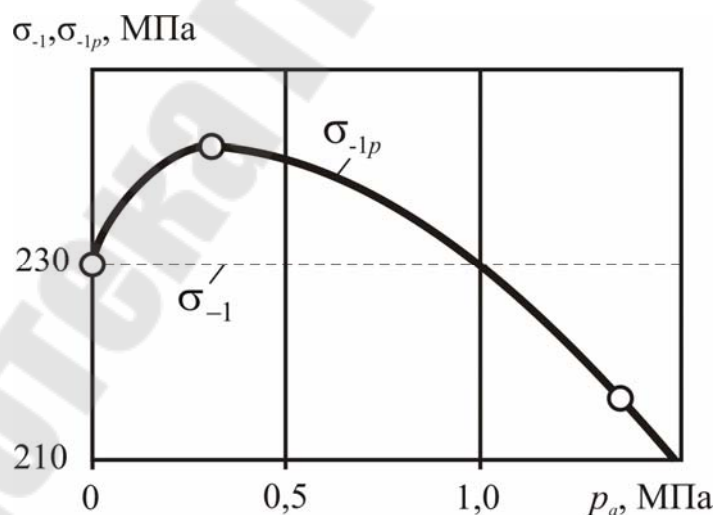
Рисунок 7.2 – Зависимость предельных напряжений от контактного давления для трибофатической системы «сталь 45 – чугун» (В. И. Похмурский и др.)
