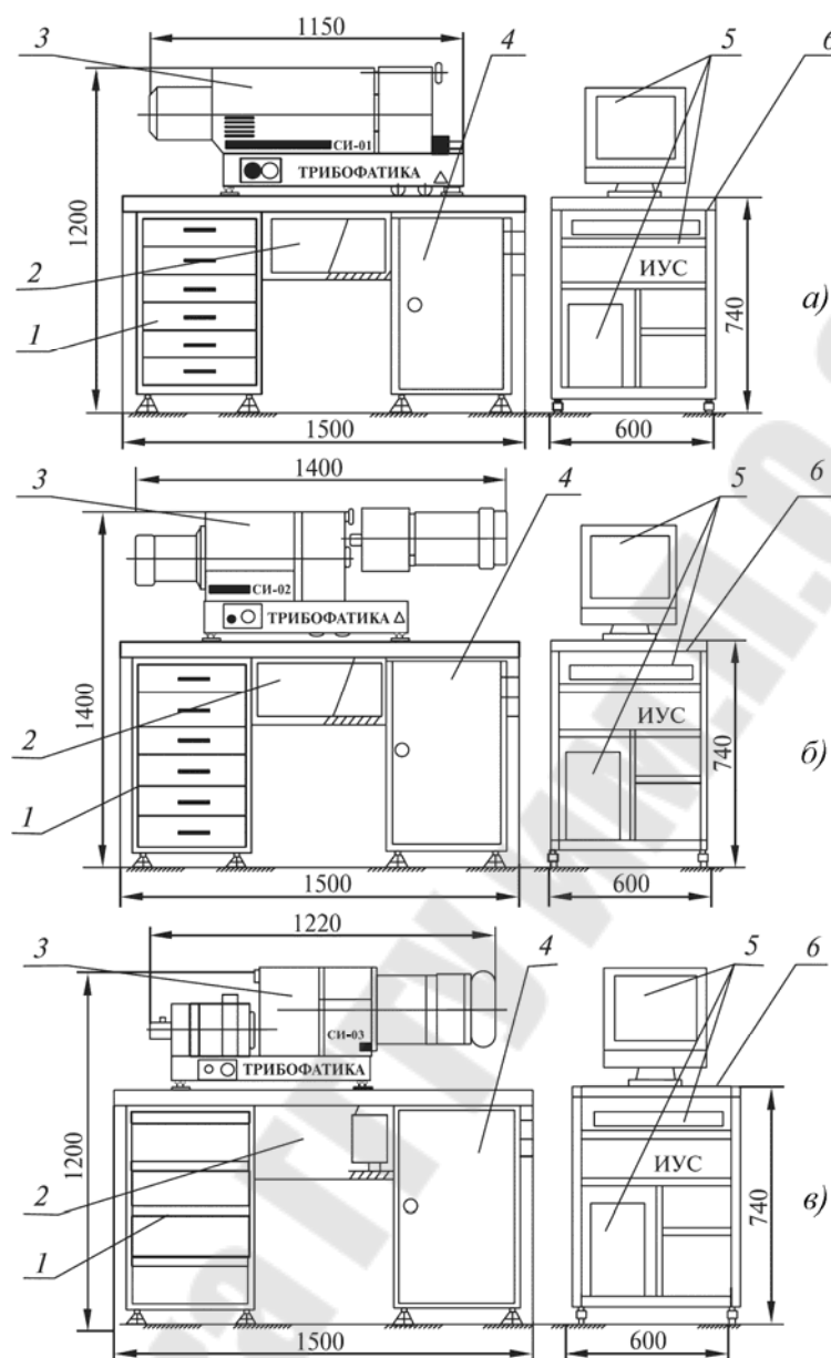
Рисунок 5.2 – Общий вид модульных машин серии СИ: а – СИ-01; б – СИ-02; в – СИ-03
