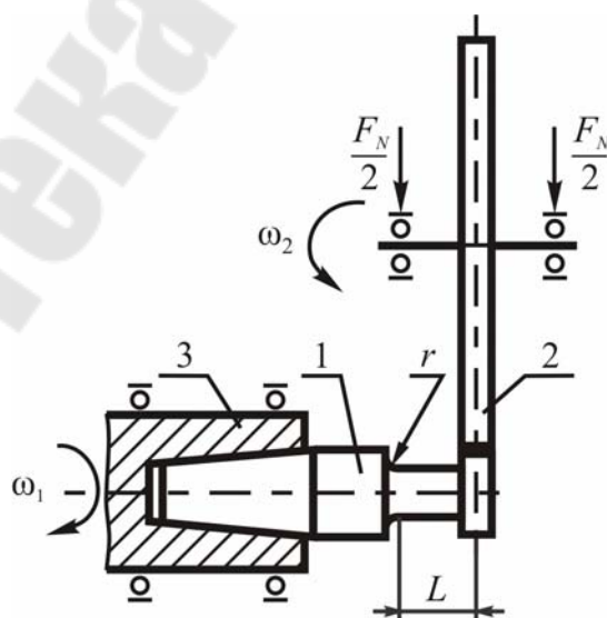
Рисунок 12.1 – Схема испытаний модели зубчатого зацепления
