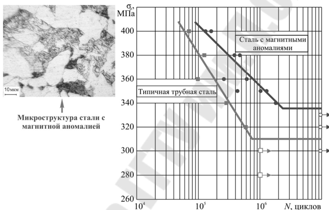
Рисунок 12.5 – Результаты испытания моделей системы «труба – поток жидкости под давлением» из типичной трубной стали и трубной стали с магнитными аномалиями
