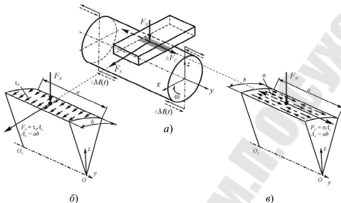
Рисунок 11.1 – Схема нагружения ТФС типа «вал – подшипник скольжения» (а) и схемы к определению однонаправленной («статической») (б) и циклической (в) составляющих силы трения в ТФС ( OO_1 – ось вала)
