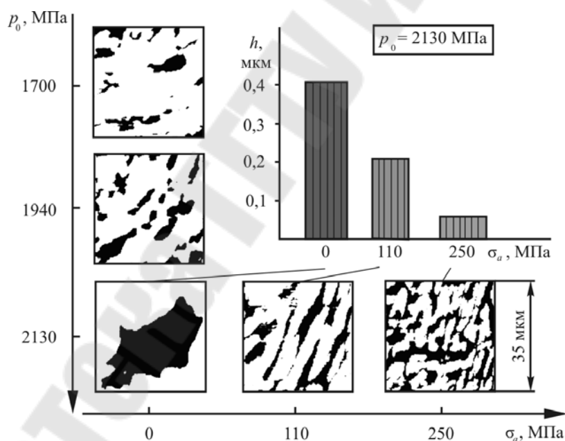
Рисунок 9.2 – Микротопографии поверхностного повреждения при трении качения (вертикальный столбец рисунков) и при износоусталостных испытаниях (остальные рисунки) (Л. А. Сосновский, С. А. Чижик и др.)
