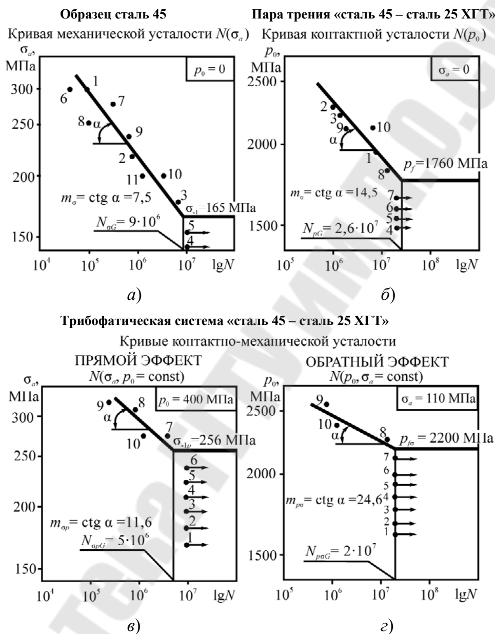
Рисунок 6.1 – К определению основных характеристик сопротивления износоусталостным повреждениям
