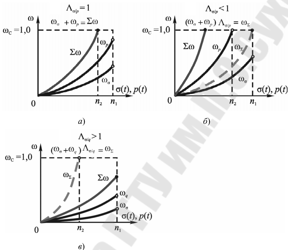
Рисунок 10.2 – Схемы, поясняющие суммирование (а) и взаимодействие (б), (в) повреждений (Л. А. Сосновский)
