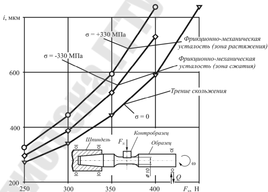
Рисунок 8.2 – Результаты износоусталостных испытаний системы «сталь 45 – полимер Ф4-ВМ» для случаев, когда трение осуществляется в зоне растяжения либо сжатия изгибаемого образца (Л. А. Сосновский, В. В. Воробьев)
