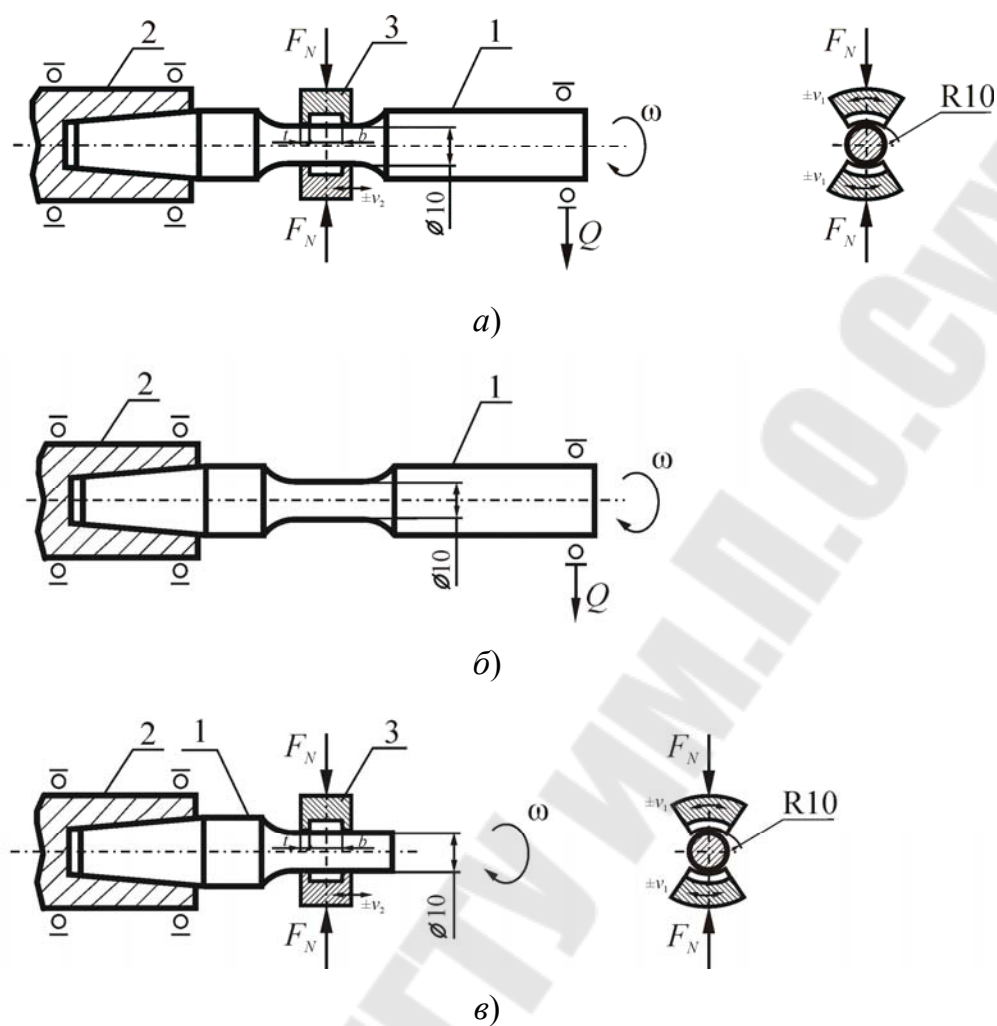
Рисунок 4.3 – Схемы испытаний на фреттинг-усталость (а), механическую усталость (б) и фреттинг (в)
