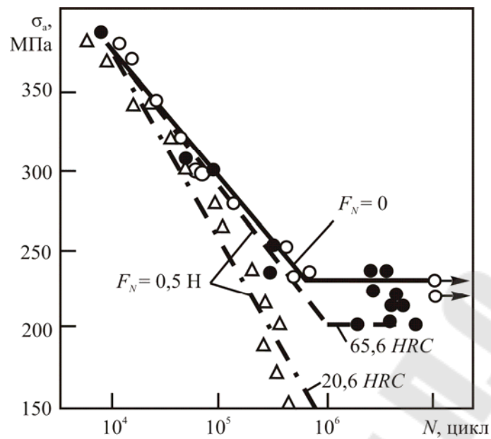
Рисунок 7.6 – Сопротивление усталости образцов углеродистой стали (0,46 % C) в зависимости от твердости HRC контртела (N. Yahata и др.)
