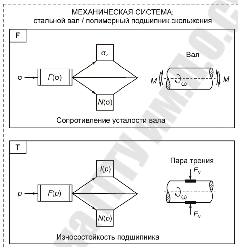
Рисунок 2.1 – Традиционный подход к расчету механической системы
