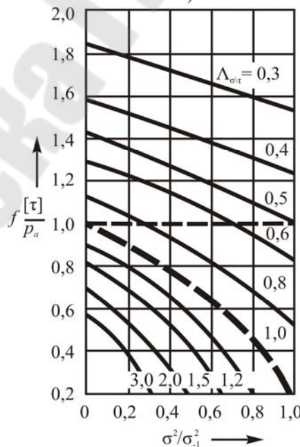
Рисунок 13.4 – К обоснованию коэффициента трения
