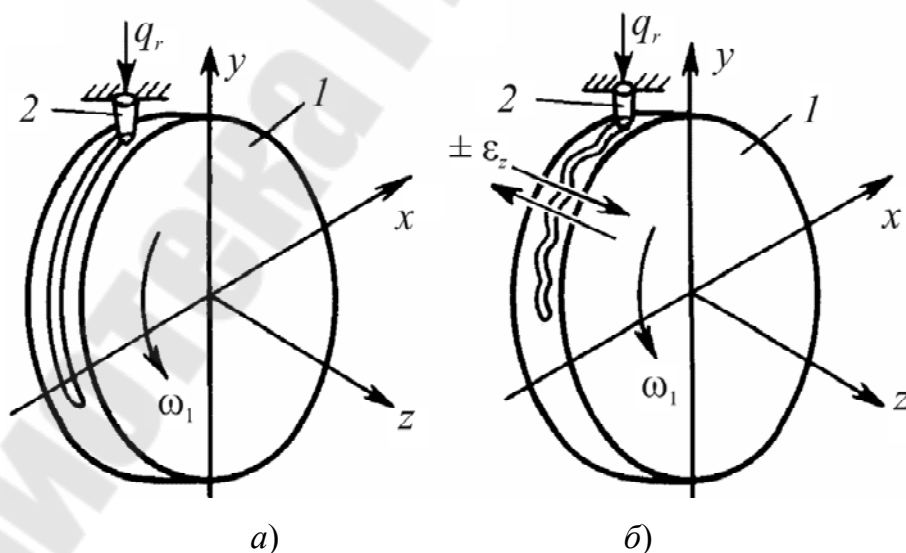
Рисунок 8.3 – К анализу обратного эффекта: а – испытания на трение; б – износоусталостные испытания
