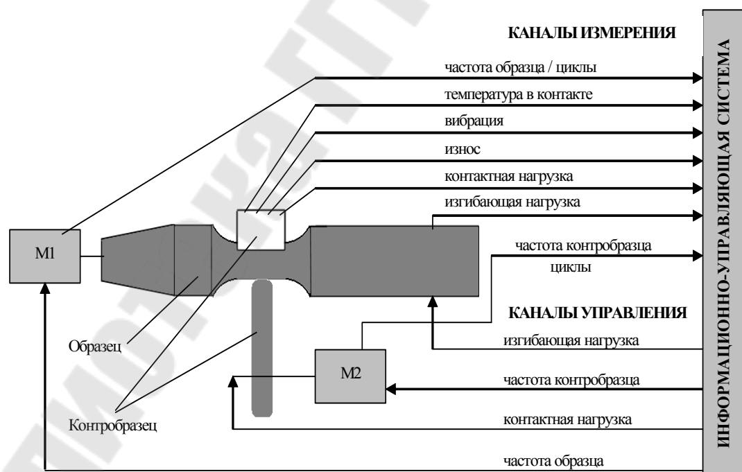
Рисунок 5.5 – Электромеханическая схема расположения датчиков в машине СИ-03: M1, M2 – приводы образца и контробразца соответственно
