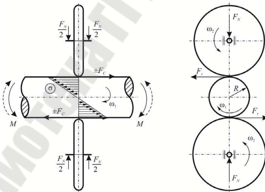
Рисунок 3.1б – Принципиальные схемы типичных трибофатических систем «твердое тело – твердое тело». Контактно-механическая усталость (КМУ)
