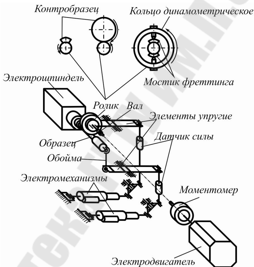
Рисунок 5.3 – Принципиальная схема испытательной установки машины СИ-03М
