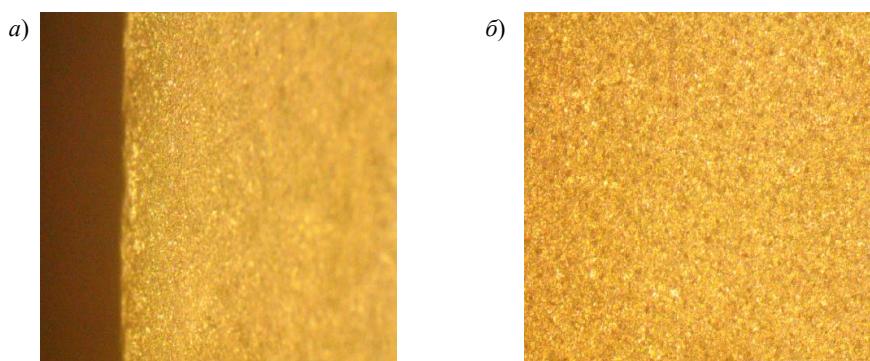
Рисунок 2 – Определение микроструктуры поверхностной зоны при увеличении 100 × (а) основного металла и при увеличении 500 × (б) с использованием тринокулярного микроскопа BS-6030
