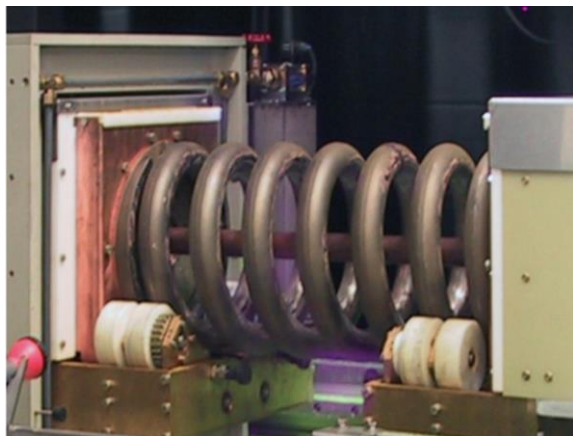
Рисунок 9 – Проведение магнитопорошкового контроля пружины с помощью дефектоскопа CRAFTST SPRING
