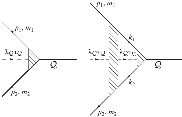
Рис. 1. Графическое уравнение для вершинной функции составной системы двух релятивистских спинных частиц произвольных масс, соответствующее правилам шпурионной диаграммной техники.
