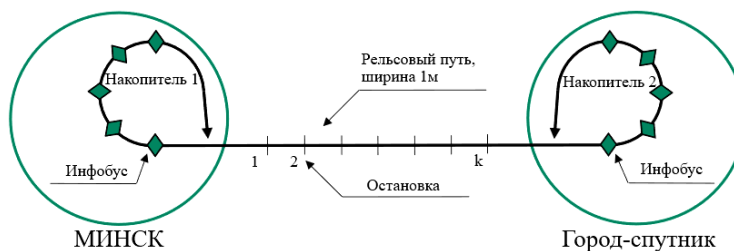
Рис. 2. Реверсная кассетно-конвейерная линия
