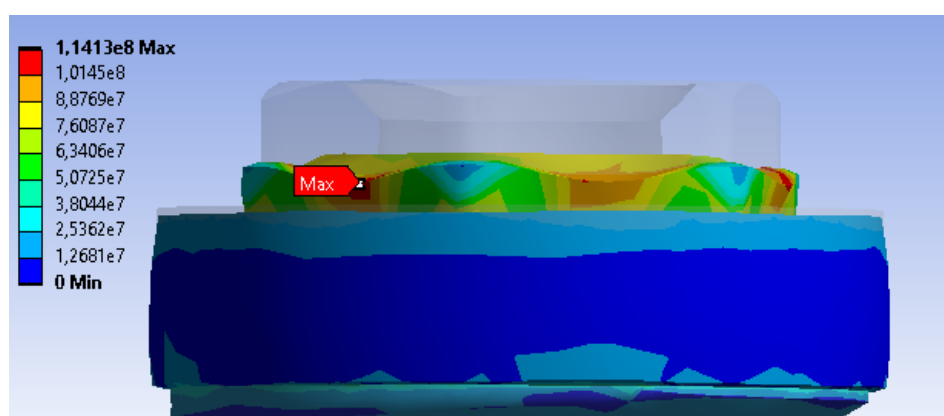
Рис. 4. Распределение напряжений имплантата
