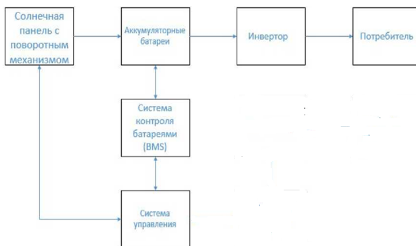
Рис. 8. Структурная схема автономного питания с использованием солнечных панелей с поворотным механизмом
