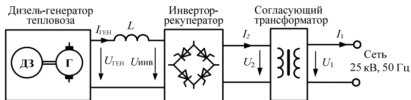
Рис. 1. Функциональная схема энергосберегающего нагрузочного устройства
