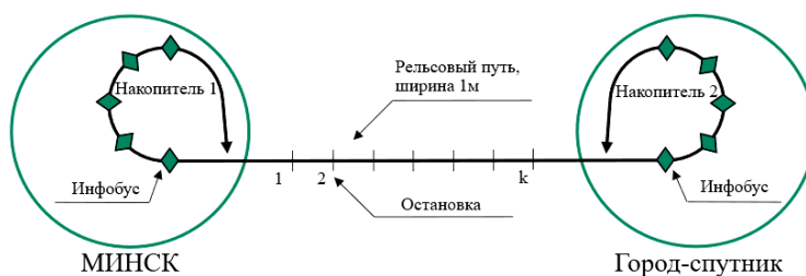
Рис. 2. Реверсная кассетно-конвейерная линия
