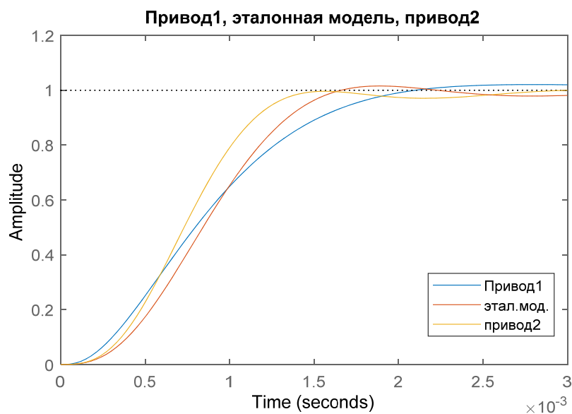
Рис. 1. Моделирование приводов
