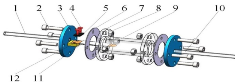
Рис. 1. Конструктивная схема пьезоэлектрического насоса с вибратором
