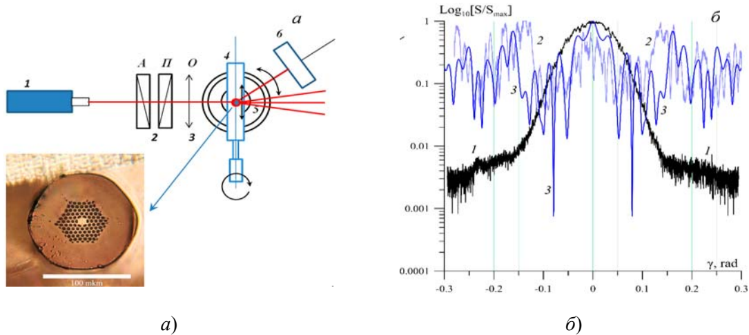
Рис. 1. Схема экспериментальной установки (а), измеренные угловые распределения интенсивности падающего гауссова пучка в перетяжке (1), пучка, рассеянного на ФКВ (2) и рассчитанное распределение интенсивности дифракционного поля (3). На вставке – снимок среза исследованного ФКВ
