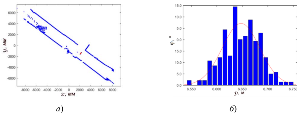
Рис. 2. Результаты тестирования RplidarA2: а – карта локализации измерений лидаром y = f(t) ; б – гистограмма распределения угла измерения от дальности \varphi = f(p)
