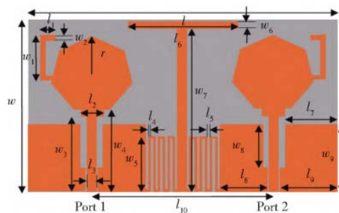
Рис. 1. Схема структуры антенны
