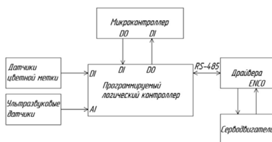
Рис. 1. Структурная схема системы автоматического управления
