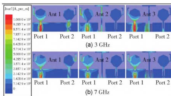
Рис. 3. Распределение электрического тока на поверхности антенны
