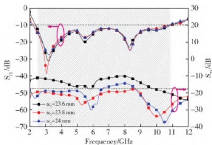
Рис. 5. Различия l_s влияние на S-параметры
