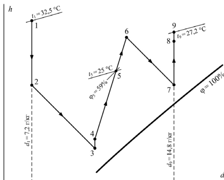
Рис. 2. Диаграмма обработки воздуха в испарительной СКВ для теплого периода года
