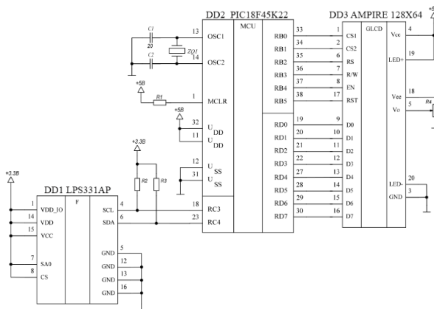
Рис. 1. Схема измерителя метеорологических параметров с графическим ЖКД
