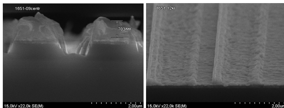
Рис. 1. РЭМ-скол SBT-пленки на монокристаллическом кремнии
