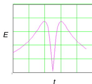
Мал. 3. Залежність сигналу на ўваходзе індукцыйнага датчыка ад часу пры руху ўнутрытрульнай кантрольна-дыягнастычнай прылады праз месца парушэння ізаляцыйнага пакрыцця нафтаправода
