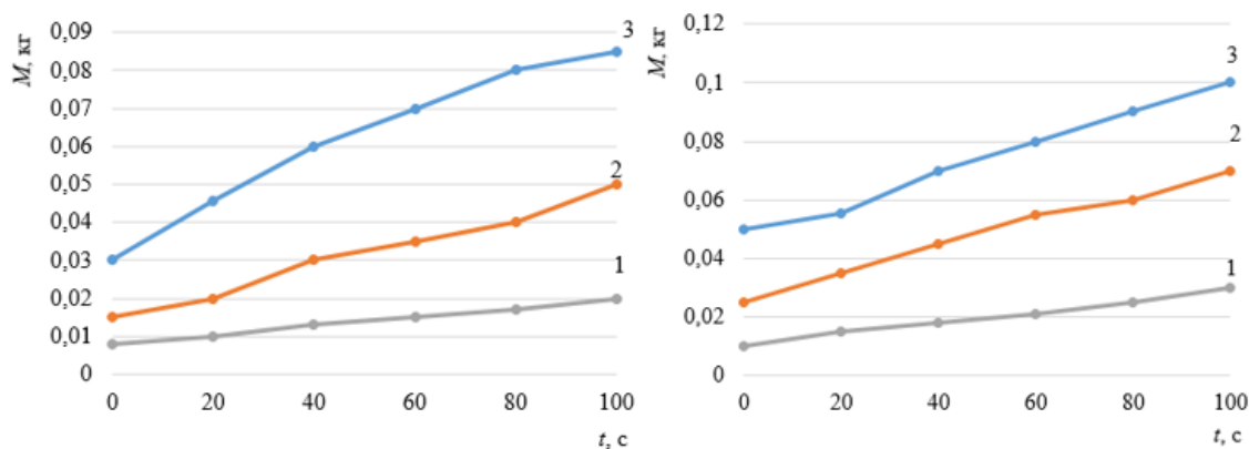
Рис. 4. Зависимость величины подачи M от времени работы устройства и угла наклона лотка устройства: ФБ-6 (315 мкм), ФБ-6 (400 мкм): 1 – угол наклона 10^\circ ; 2 – угол наклона 30^\circ ; 3 – угол наклона 50^\circ
