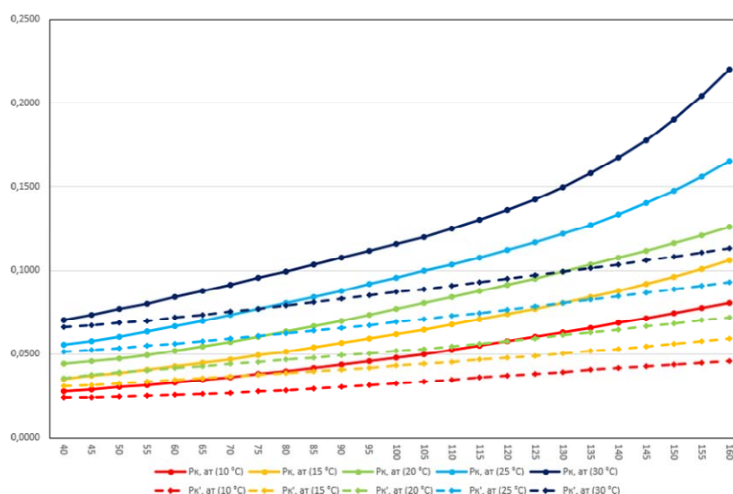
Рис. 2. Зависимость давления в конденсаторе от пропуски пара в конденсатор при различных температурах охлаждающей воды: — — — — при одном включенном насосе, — — — — при двух включенных насосах
