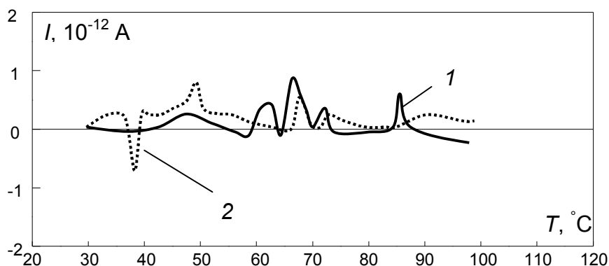
Рисунок 1 – Спектры ТСТ оливкового масла (усреднение по шести повторам) (1 – исходный образец; 2 – образец после термообработки)
