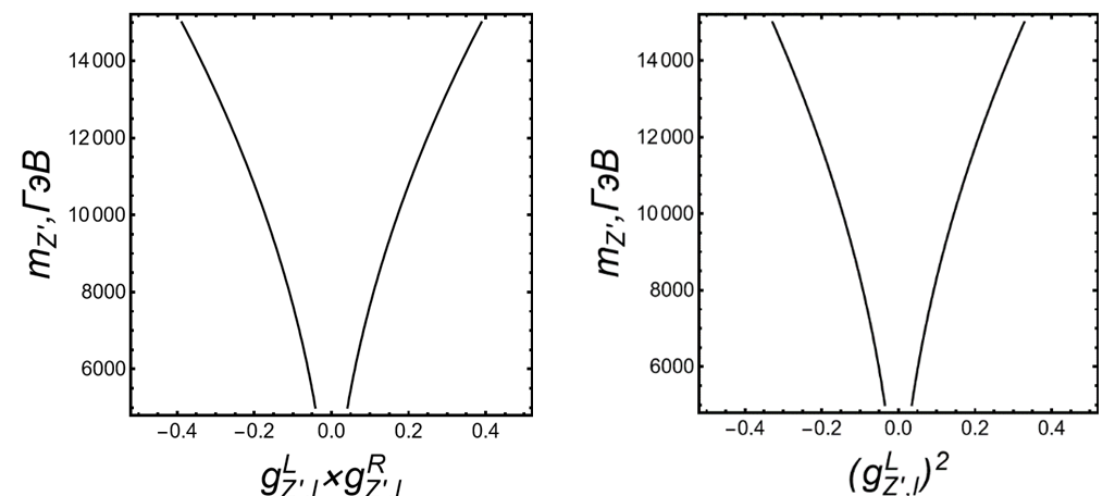
الشكل 1- القيود على m_{Z'} و g_{Z',l}^{\lambda_e} \times g_{Z',l}^{\lambda_{\tau}} لعملية e^+e^- \rightarrow \tau\bar{\tau} - مروحية الحالات الأولية والنهائية، على التوالي)
