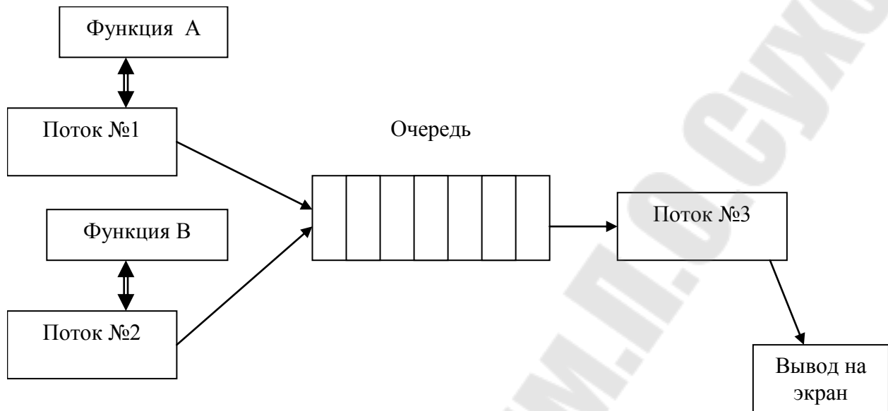
Рис. 1 – Схема многопоточного приложения
