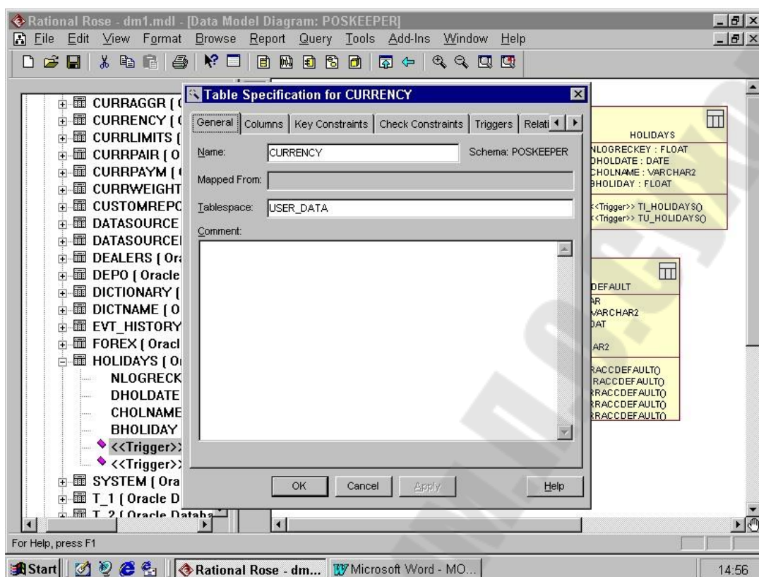
Рисунок 5.2 - Окно спецификации таблицы
