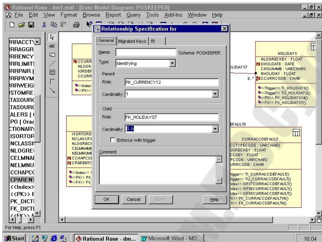
Рисунок 5.3 - Окно спецификации связи
