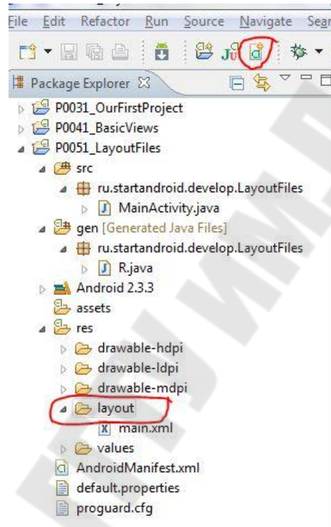
Рисунок 2.1 – Создание layout-файла
