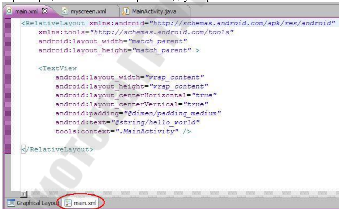
Рисунок 4.1 – Файл main.xml
