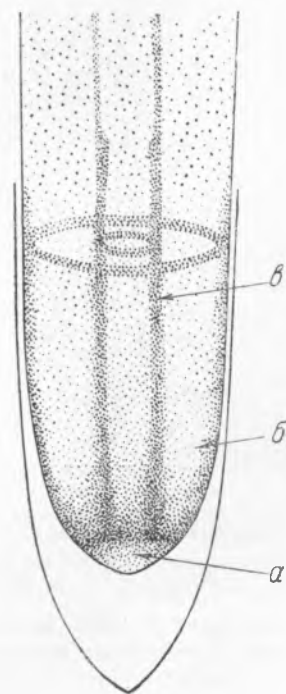
Рис. 1. Схема распределения базофильных клеток в корешке у покрытосемянных растений: а — группа инициальных клеток; б — наружный базофильный цилиндр; в — внутренний базофильный цилиндр. Вверху цилиндрические слои изображены в поперечном разрезе
