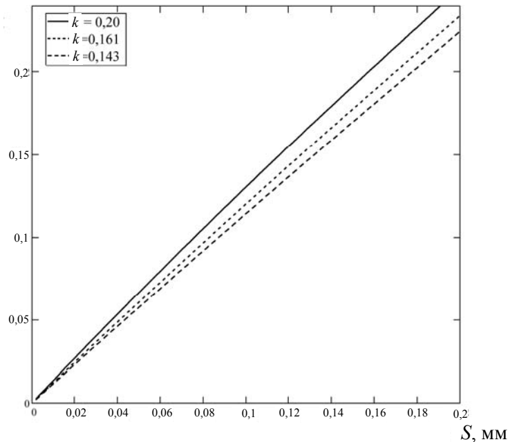
Рис. 2. Номограмма для определения размера области распространения тепла от точечного источника на поверхность проволоки диаметром d_{п} = 0,3 мм в зависимости от величины межэлектродного промежутка при различных соотношениях k
