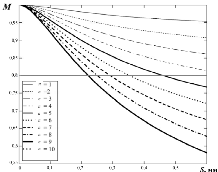
Рис. 4. Изменение относительной площади M поперечного сечения обработанной проволоки при различных количествах сторон обработки в зависимости от величины межэлектродного промежутка
