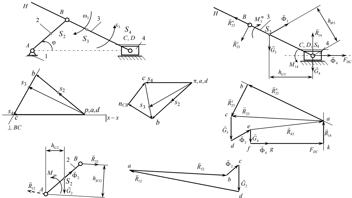
Рис. 1. План положений, план скоростей, план ускорений и силовой анализ плоского рычажного механизма
