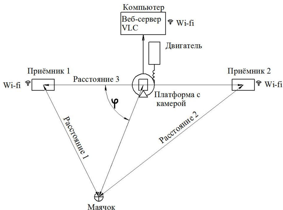
Рис. 1. Схема системы наведения видеокамеры
