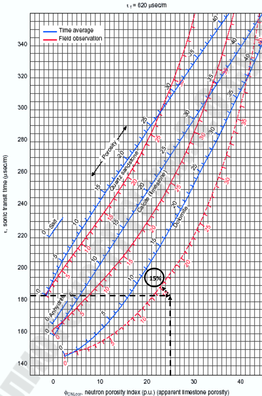
Рис. 3.1. Палетка для определения пористости и литологии по акустическому (sonic transit time) каротажу и нейтронному методу пористости (neutron porosity index)
