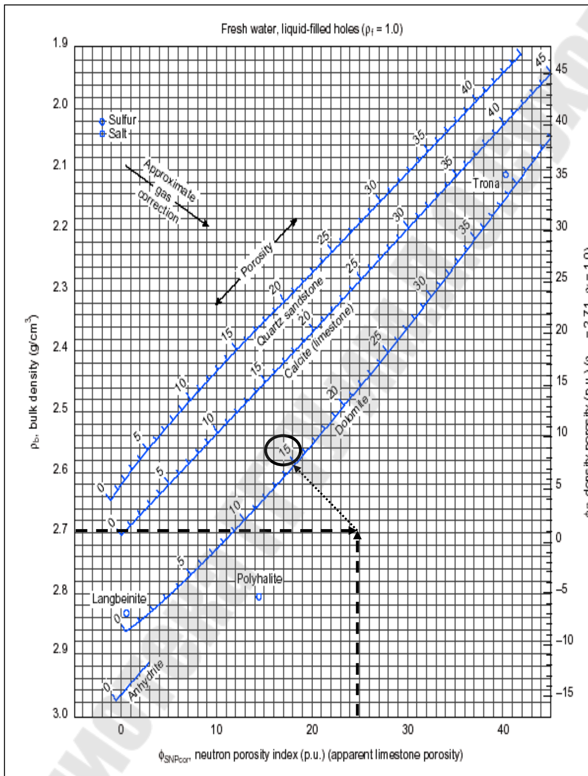
Рис. 3.2. Палетка для определения пористости по плотностному (bulk density) каротажу и нейтронному методу пористости (neutro porosity index).
