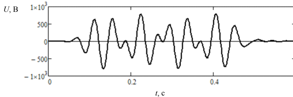
Рис. 3. Сигнал на выходе фильтра
