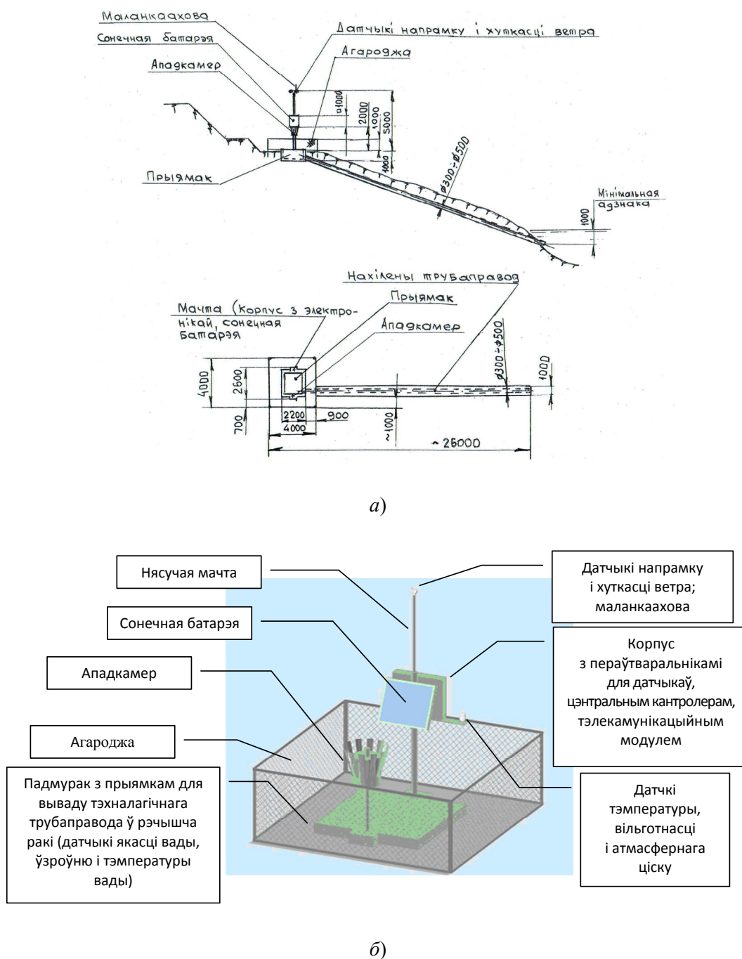
Мал. 2. Канструктыўная кампануўка (а) і папярэдняя 3D-мадэль канструкцыі (б) станцыі AHMES
