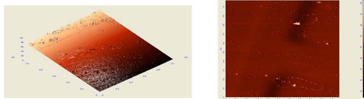
Рис. 1. АСМ-изображение и распределение фаз поверхности пленки, приготовленной на основе тетраэтилортосиликата
