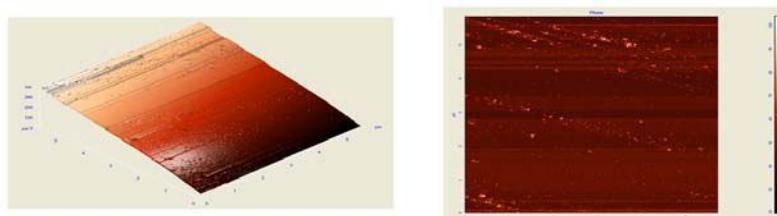
Рис. 2. АСМ-изображение и распределение фаз поверхности пленки, приготовленной на основе винилтриэтоксисилана
