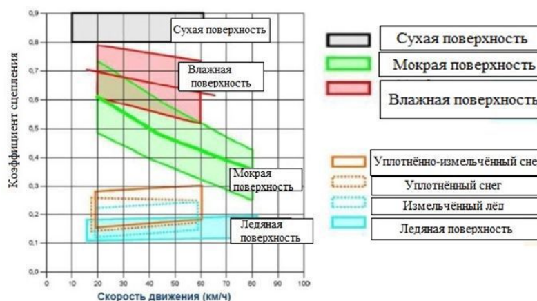
Рис. 3. Коэффициент сцепления при различных дорожных условиях
