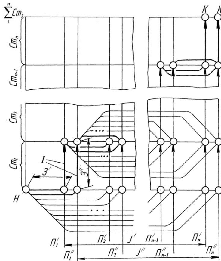
Рис. 5. Схема модели двухпараметрической оптимизации состава однотипного технологического оборудования ремонтного завода:
