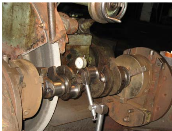
Рис. 1. Измерение смещения оси обрабатываемой шейки коленчатого вала от оси вращения шпинделя станка
