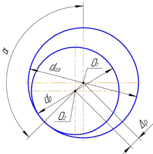
Рис. 2. Схема расположения контура шатунной шейки вала после обработки диаметром d_p в контуре шейки до обработки диаметром d_{из} : O_1 – центр окружности изношенной шейки; O_2 – центр окружностей, совпадающий с осью вращения шпинделя станка; \alpha – угол между линией центров окружностей и осью кривошипа; \Delta_p – геометрическая сумма отклонений расположения и формы обрабатываемой поверхности
