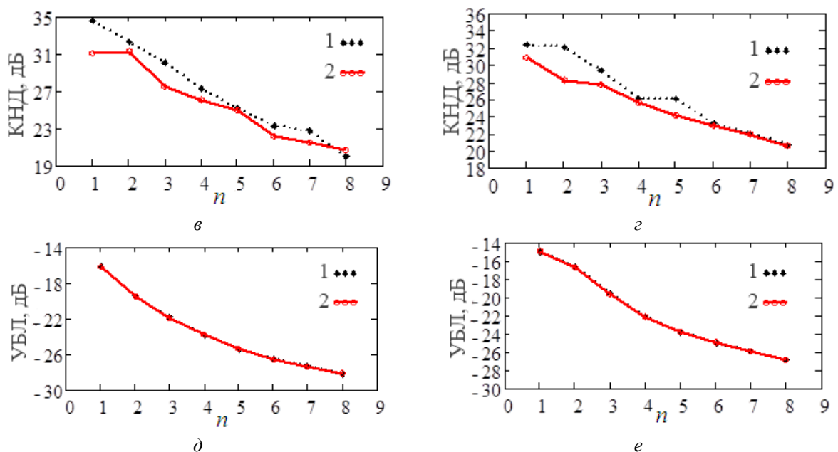
Рис. 5. Выходные характеристики двух АР для разных распределений амплитуд
