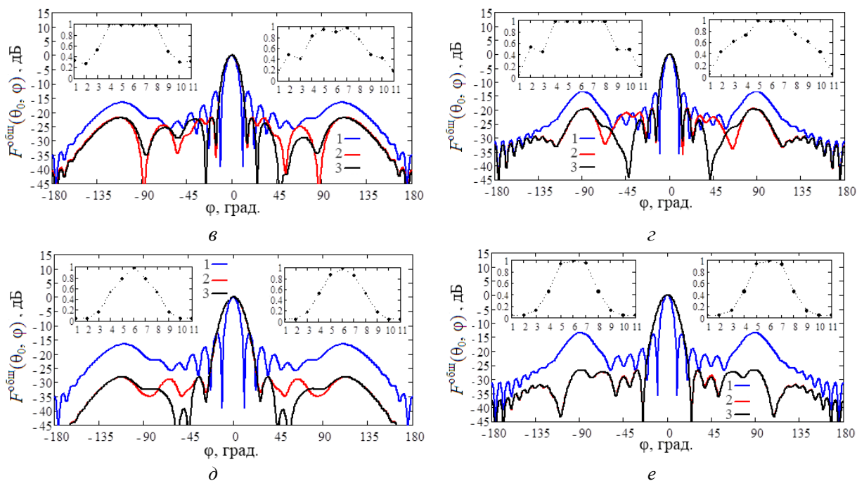
Рис. 4. ДН двух типов АР при разных амплитудных распределениях синтезированных двумя методами PSO
