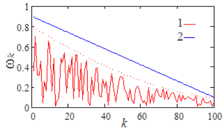
Рис. 1. Зависимость весового коэффициента от номера итерации
