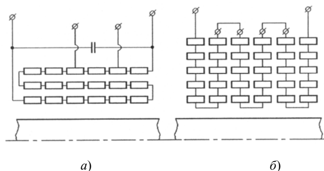
Рис. 1. Схемы многослойных индукторов
