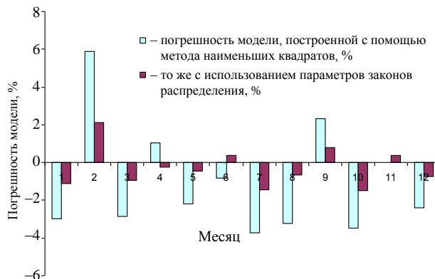
Рис. 7. Динамика погрешностей моделей при прогнозе месячного потребления ЭЭ
