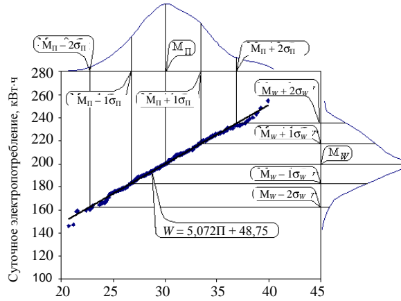
Рис. 5. Построение модели потребления ЭЭ с использованием параметров законов распределения объемов выпускаемой продукции и расхода электрической энергии
