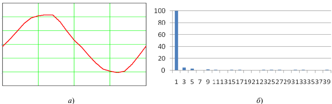
Рис. 1. Экспериментальная кривая тока индукционных световых приборов типа 03-022 с индукционной лампой мощностью 150 Вт и гармонический состав кривой тока ( K_{\text{нс}} = 6,12\% )
