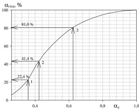
Рис. 3. Доля годового расхода теплоты, покрываемая тепловыми насосами комбинированной теплонасосной станции при \tau_{\text{ТНУ}_{\text{max}}} = 70^\circ\text{C} для температурных графиков: 1 – 150/70 ^\circ\text{C} ; 2 – 130/70; 3 – 95/70 ^\circ\text{C}
