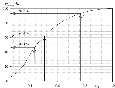
Рис. 4. Доля годового расхода теплоты, покрываемая тепловыми насосами комбинированной теплонасосной станции при \tau_{\text{ТНУ}_{\text{max}}} = 80^\circ\text{C} для температурных графиков: 1 – 150/70 ^\circ\text{C} ; 2 – 130/70; 3 – 95/70 ^\circ\text{C}
