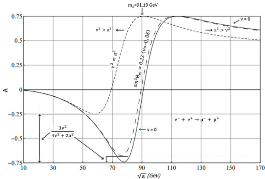
Рисунок 2 – Зависимость аналогичная графикам, приведенным на рисунке 1, но для асимметрии вперед-назад A_{FB}
