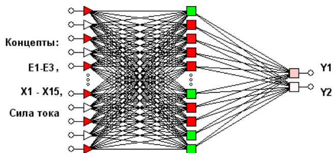
Рис. 3. Архитектура нейросетевой (многослойный перцептрон) оценки сценарно-когнитивного моделирования
