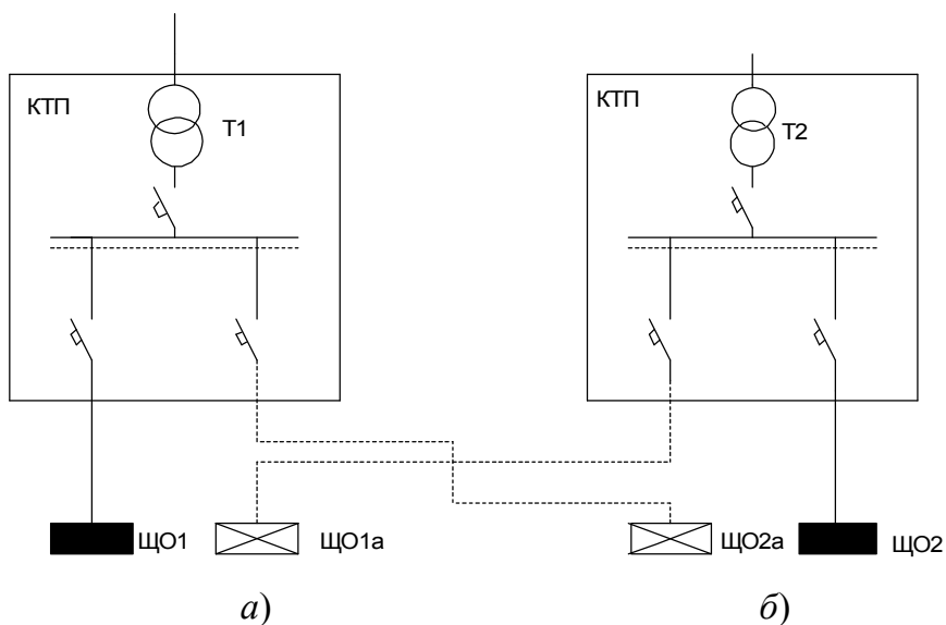
Рис. 3.7. Схема питания электрического освещения от двух однотономных подстанций
