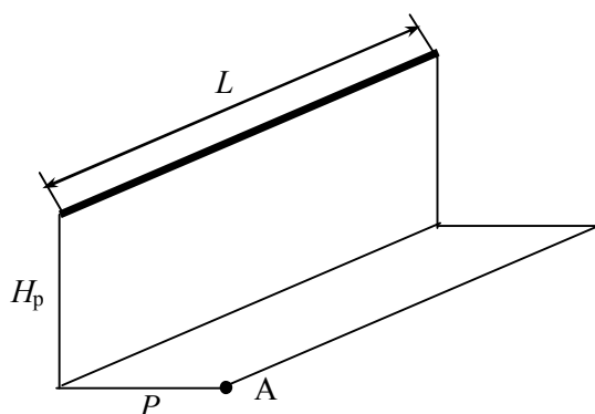
Рис. 2.5. Светящая линия ( L ) с указанием размеров, определяющих положение ее по отношению к контрольной точке; H_p – расчетная высота подвеса светильников; p – расстояние от контрольной точки в плоскости, перпендикулярной светящей линии до перпендикуляра, опущенного на расчетную плоскость от светящей линии
