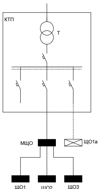
Рис. 3.9. Схема питания групповых щитков от магистрального щитка
