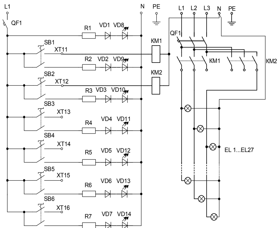
Рис. 4.2. Фрагмент схемы электрической принципиальной дистанционного управления с помощью электромагнитных пускателей
