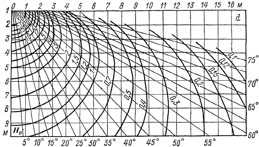
Рис. 2.3. Пространственные изолюксы условной горизонтальной освещенности. Сила света светильника по всем направлениям 100 кд
