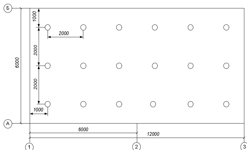
Рис. 2.1. Размещение светильников на плане помещения
