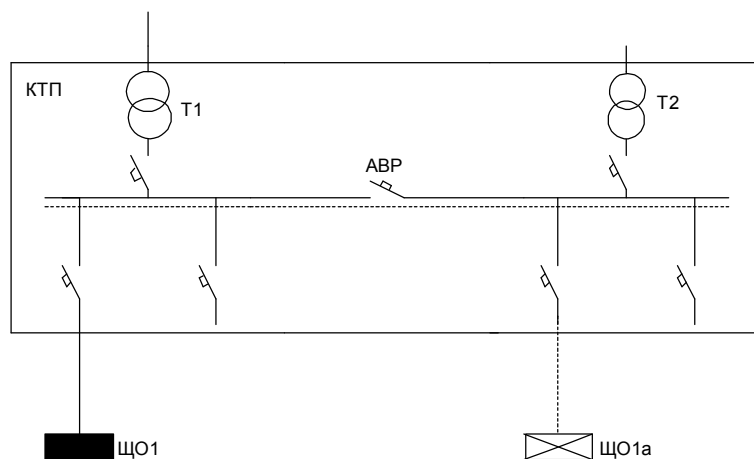
Рис. 3.8. Схема питания электрического освещения от двухтрансформаторной подстанции
