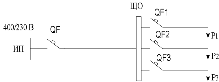
Рис. 3.11. Схема к задаче 3.6
