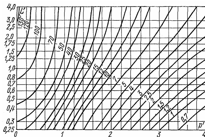
Рис. 2.6. Линейные изолюксы для светильников ЛПП
