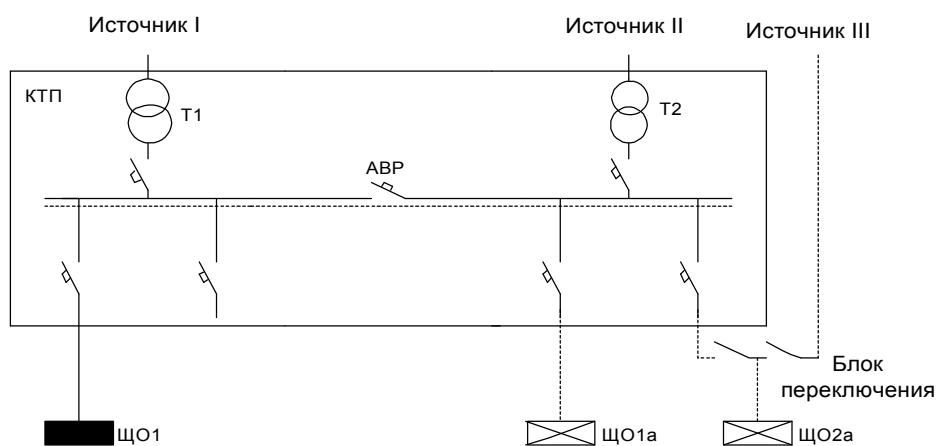
Рис. 3.10. Схема питания электрического освещения от трех источников
