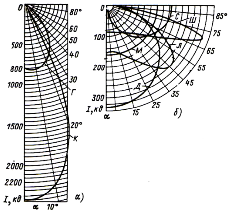
Рис. 1.2. Типовые кривые силы света светильников
