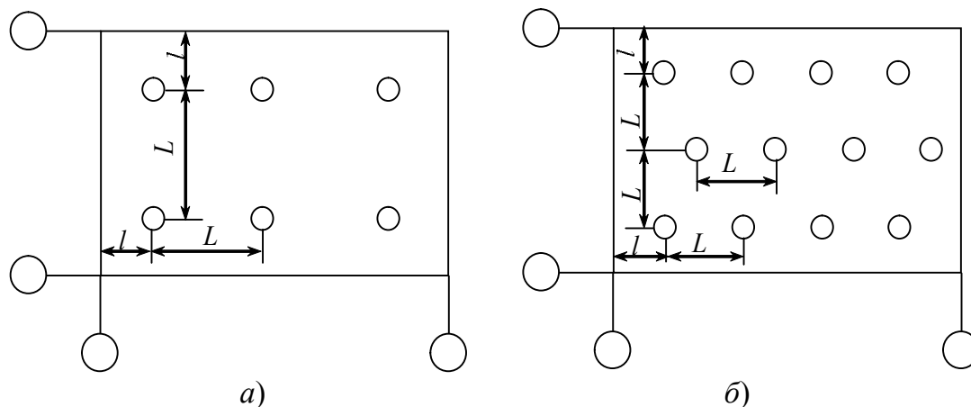
Рис. 1.4. Размещение светильников на плане помещения: а – по углам прямоугольника; б – в шахматном порядке
