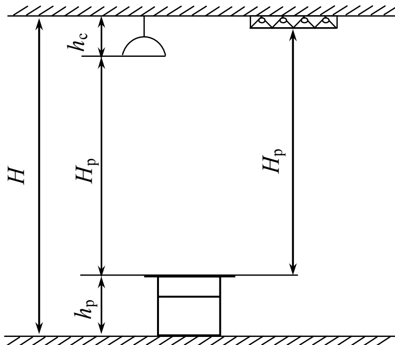
Рис. 1.3. Размещение светильников по высоте помещения
