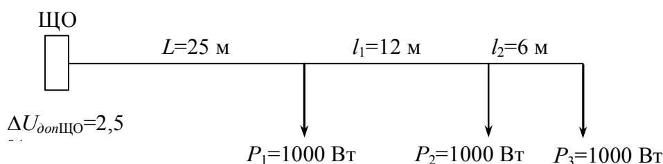
Рис. 3.2. Схема к задаче 3.3
