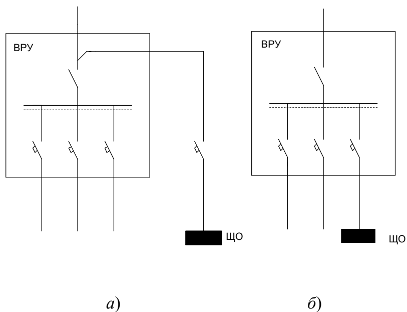
Рис. 3.5. Схема питания электрического освещения от вводно-распределительного устройства
