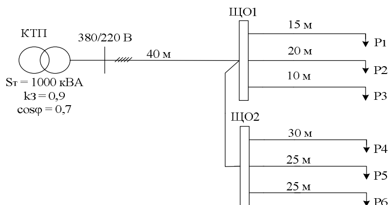
Рис. 3.4. Схема к задаче 3.5
