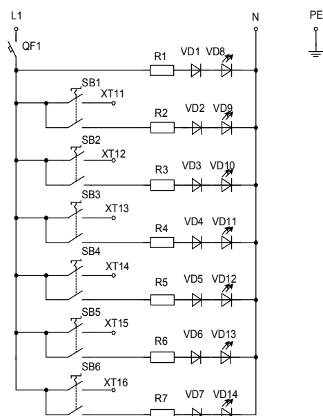
Рис. 4.1. Схема электрическая принципиальная пульта дистанционного управления
