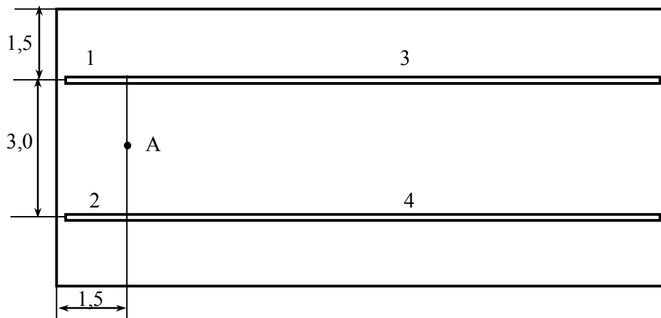
Рис. 2.7. Схема к расчету освещенности в точке А
