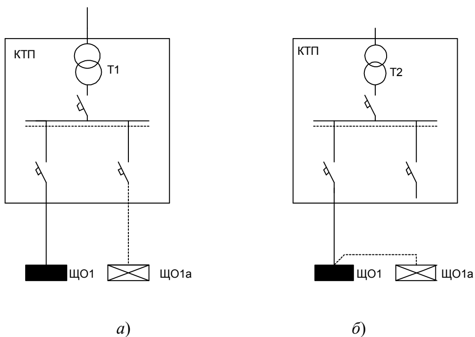
Рис. 3.6. Схема питания освещения от однострансформаторной подстанции
