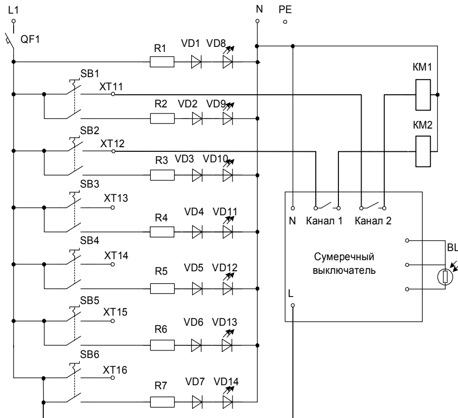
Рис. 4.3. Схема автоматического управления осветительной установкой внутреннего освещения
