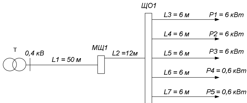
Рис. 3.3. Схема к задаче 3.4
