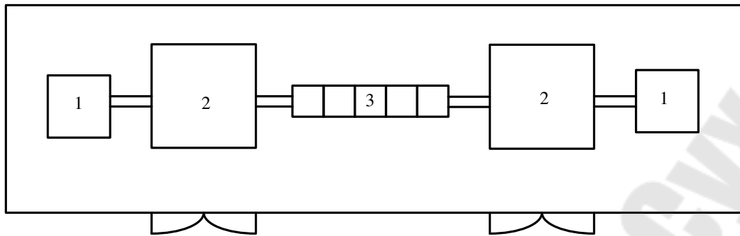
Рис. 6.3 – Однорядное расположение двухтрансформаторной подстанции
