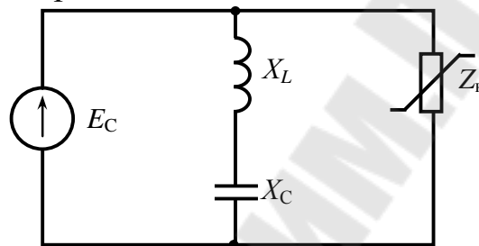
Рис. 17.7 – . Схема замещения силового резонансного фильтра
