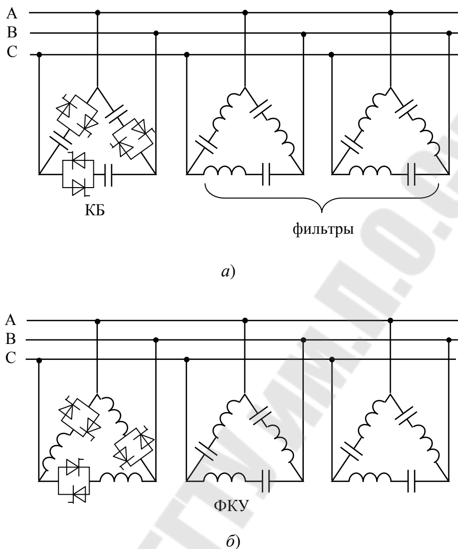
Рис. 17.8 - Структурные схемы многофункциональных ИРМ прямой (а) и косвенной (б) компенсации
