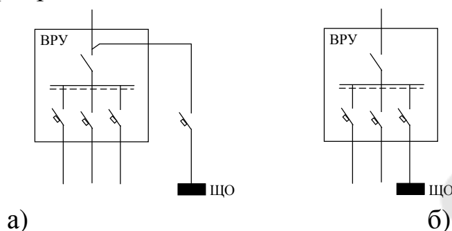
Рис. 2.10 – Схема питания ОУ от ВРУ
