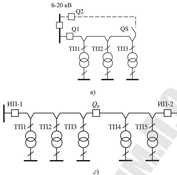
Рис. 5.2 – Магистральные схемы внутриводского электроснабжения: а – однониточная магистральная схема; б – схема двойной сквозной магистрали; в – однониточная магистральная схема с резервной перемычкой; г – магистральная схема с двухсторонним питанием
