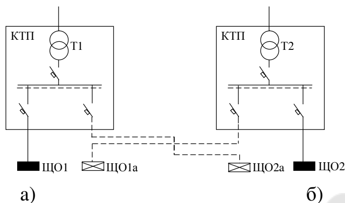
Рис. 2.12 – Схема питания ОУ от двух однострановторных подстанций
