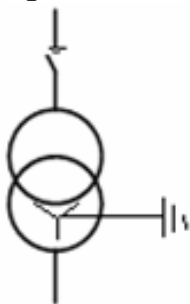
Рис. 5.6 – Схема присоединения трансформатора через выключатель нагрузки
