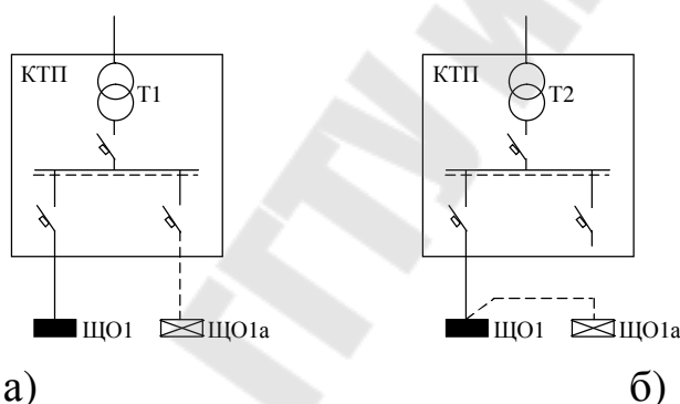
Рис. 2.11 – Схема питания рабочего и аварийного освещения от однострансформаторной подстанции
