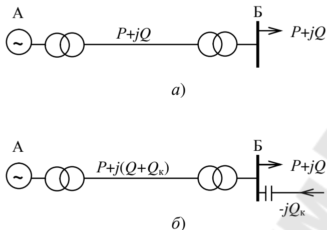
Рис. 10.4 – Схемы электропередачи: а – без компенсации;
