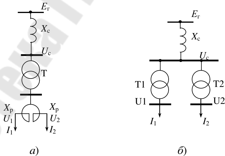
Рис. 17.3 – Разделение нагрузок с помощью сдвоенного реактора (а) и различных трансформаторов (б)
