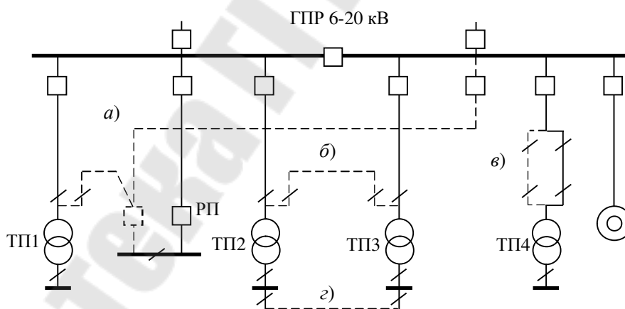
Рис. 5.1 – Схема радиального питания: а – резервная магистраль высокого напряжения; б – резервная связь на стороне высшего напряжения между ТП; в – резервная линия высокого напряжения; з – резервная связь на стороне до 1 кВ между ТП или токопроводами
