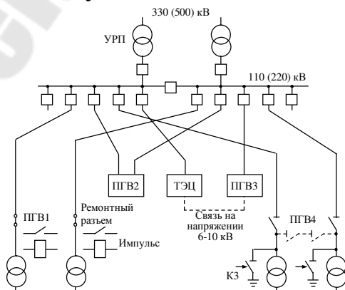
Рис. 4.6 – Радиальная схема электроснабжения при системе глубоких вводов 110-220кВ
