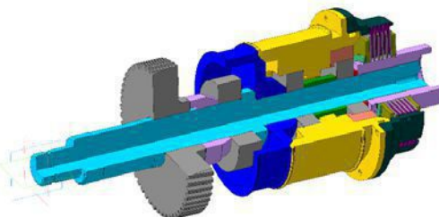
Рис. 1. Трехмерная модель узла натяжения сдвоенного кабестана
