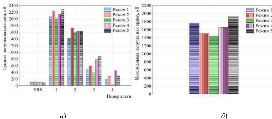
Рис. 1. Средние нагрузки, действующие на прокатный инструмент:
