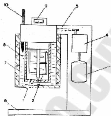
Рис.52. Схема консистометра КЦ-5
