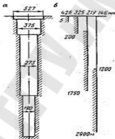
Рис. 2. Пример профиля (а) и рабочей схемы (в) конструкции скважины
