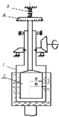
Рис. 34. Схема ротационного вискозиметра:
