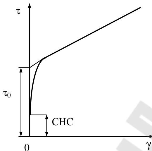
Рис. 20. Реограмма вязкопластичных жидкостей
