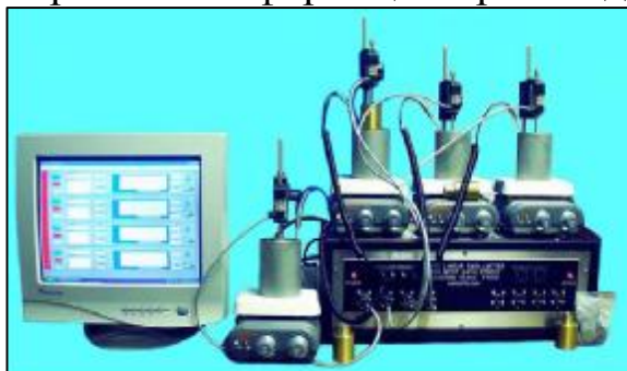
Рис.42. Тестор ингибирующей способности OFITE
