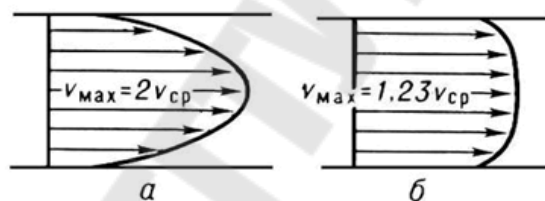
Рис.24. Профиль осреднённой скорости: а — при ламинарном, б — при турбулентном течении.
