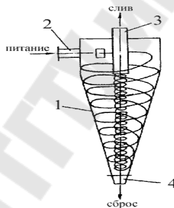
Рис. 10. Схема гидроциклона
