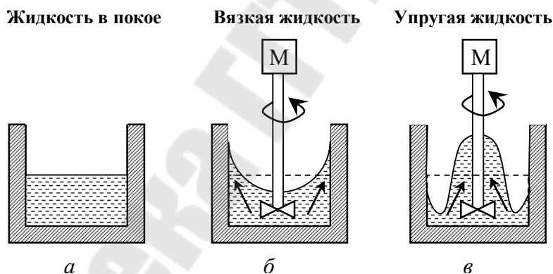
Рис. 55. Реакция на сдвиг вязкой и упругой жидкостей
