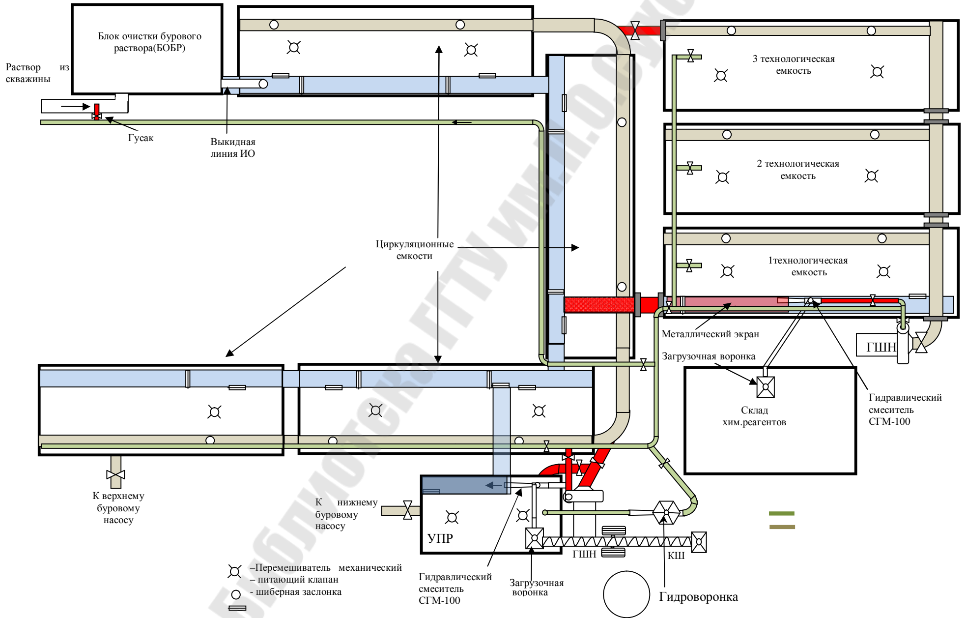
Рис.5. Принципиальная схема обвязки оборудования для приготовления и обработки БР
