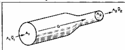
Рис.25. Непрерывность потока: скорость жидкости обратно пропорциональна площади поперечного сечения в направлении потока
