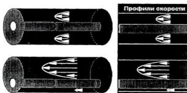
Рис.45. Влияние эксцентрического расположения труб на скорость бурового раствора в затрубном пространстве
