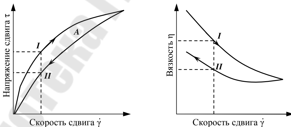
Рис.21. Кривые вязкости и пластичности, описывающие явление тиксотропии
