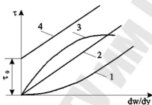
Рис.19. Реограммы жидкостей: 1- дилатантной ( n < 1 ); 2- ньютоновской ( n = 1 ); 3- псевдопластичной ( n > 1 ); 4- вязкопластичной;
