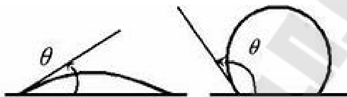
Рис. 14. Гидрофильная и гидрофобная поверхности
