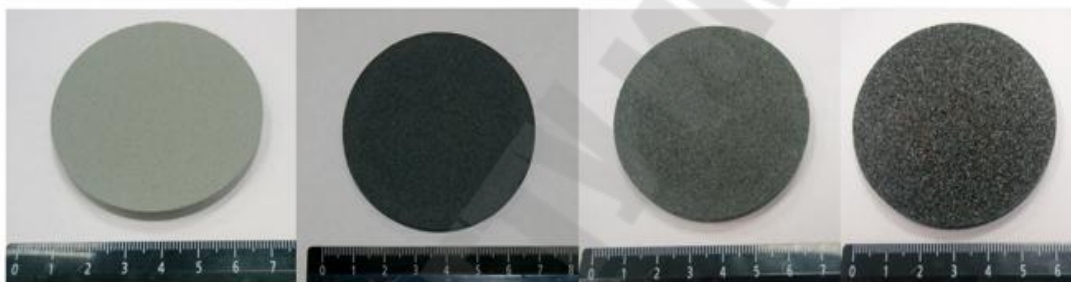
Рис.49. Керамические диски с проницаемостью (слева направо) 10, 20, 35, 90 мкм производства OFITE, используемые в качестве пористой среды
