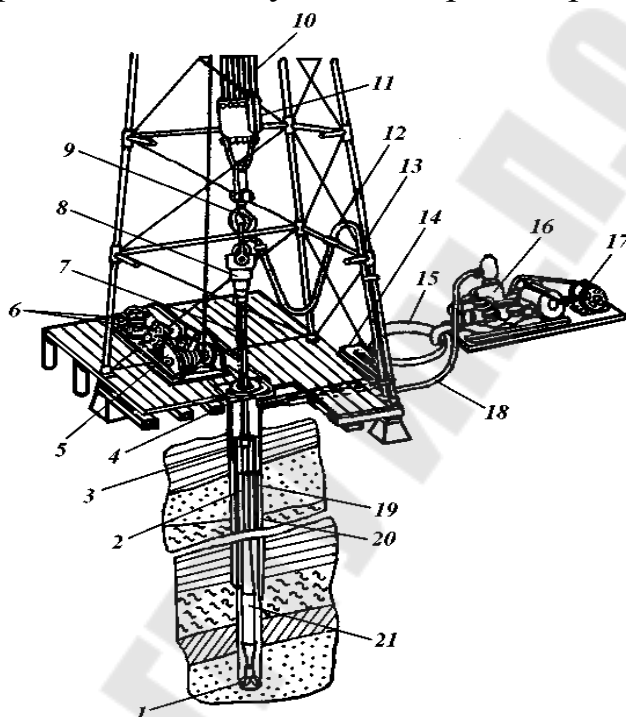
Рис. 1. Схема бурения скважины:
