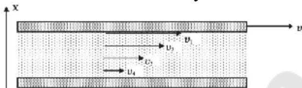
Рис.16. Течение вязкой жидкости между пластинами
