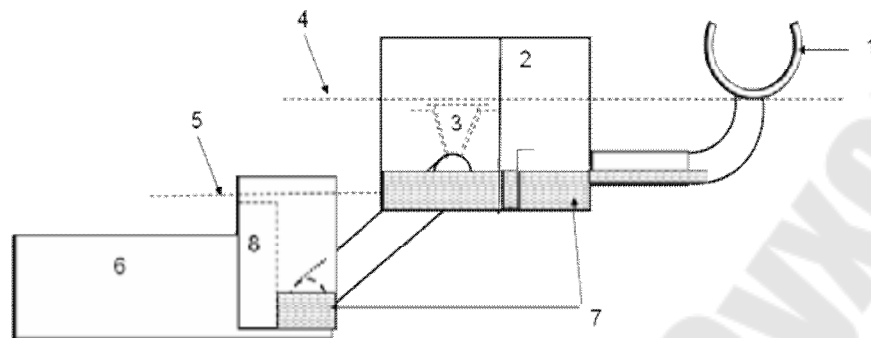
Рис.8. Подключение распределителя потока бурового раствора к желобной системе и виброситам 1-желоб; 2 - распределитель потоков; 3 - заслонка; 4 - граница перелива через заслонку; 5 - линия водослива вибросита; 6 - вибросито; 7 - зоны накопления шлама; 8 – питатель вибросита.
