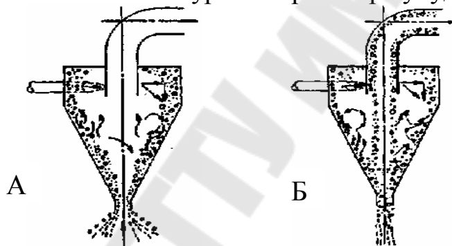
Рис. 11. Разгрузка гидроциклона веером А и шнуром Б
