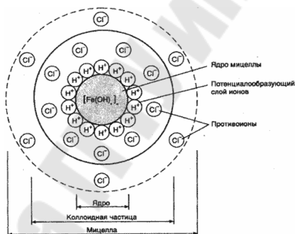
Рис.13. Строение коллоидной мицеллы
