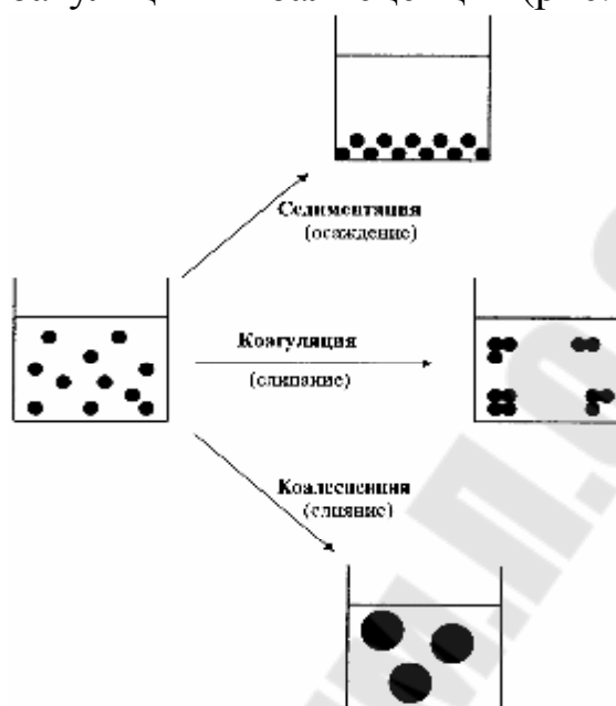
Рис.15. Процессы, вызывающие потерю устойчивости дисперсных систем
