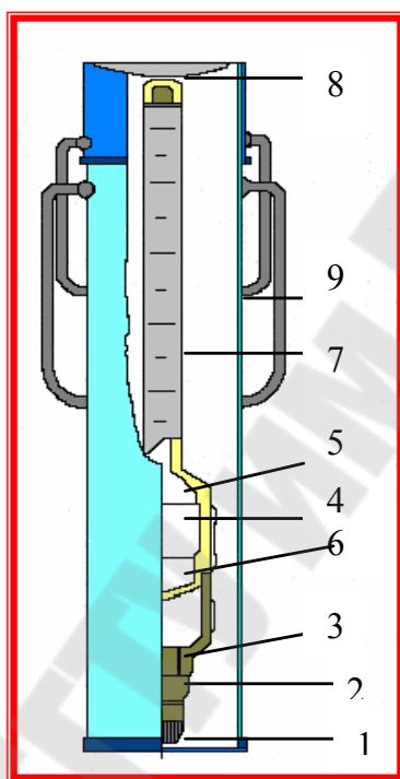
Рис.2.1. Ареометр АБР-1: 1 – съемный груз; 2 – полиэтиленовая заглушка; 3 – металлический балласт; 4 – мерный стакан; 5 – крышка поплавка; 6 – дношко поплавка; 7 – стержень с нанесенными на нем основной и поправочной шкалами; 8 – пробка; 9 – ведро
