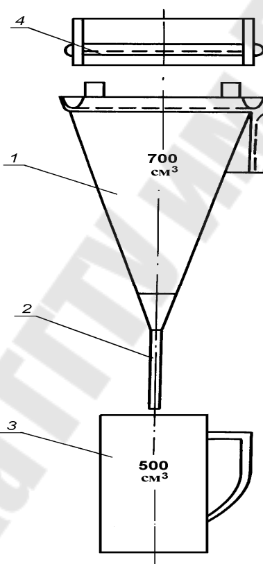
Рис.2.3. Вискозиметр ВБР-1
