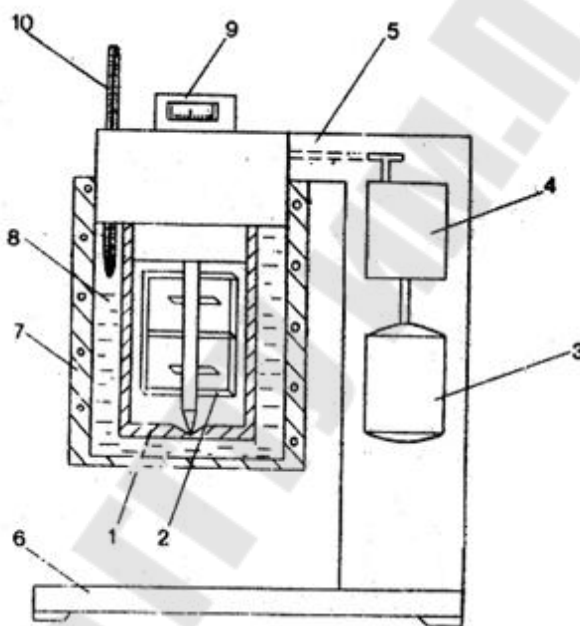
Рис.4.9. Схема консистометра КЦ-3: 1-стакан для раствора; 2-рамка с лопастями; 3-электродвигатель; 4-редуктор; 5- кронштейн; 6- станина; 7 - электронагреватель; 8- водяная баня;9- шкала; 10- термометр
