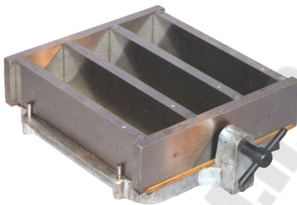
Рис.4.3. Форма для изготовления цементных балочек размером 4x4x16 см
