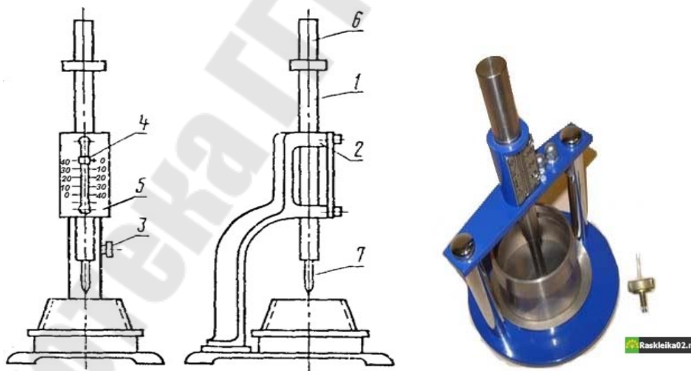
Рис.4.1. Схема и прибор «Игла Вика» ИВ-2: 1 - цилиндрический металлический стержень; 2 - обойма станины; 3 - стопорное устройство; 4 - указатель; 5 - шкала; 6 - пестик; 7 - игла
