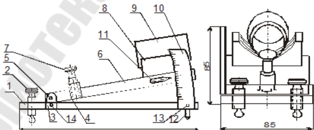
Рис.3.7. Прибор для определения коэффициента трения фильтрационной корки бурового раствора КТК-2
