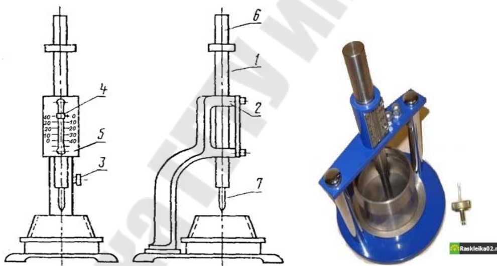
Рис.2.7. Схема и прибор «Игла Вика» ИВ-2: 1 - цилиндрический металлический стержень; 2 - обойма станины; 3 - стопорное устройство; 4 - указатель; 5 - шкала; 6 - пестик; 7 - игла
