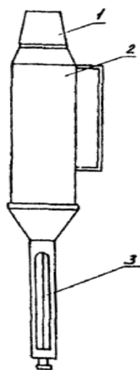
Рис.3.9. Металлический отстойник ОМ-2: 1-крышка, 2-отстойник, 3-стеклянная бюретка
