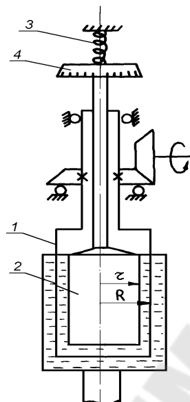
Рис.3.1. Общая схема ротационного вискозиметра: 1 – наружный вращающийся цилиндр; 2– внутренний вращающийся цилиндр; 3 – пружина; 4 – шкала
