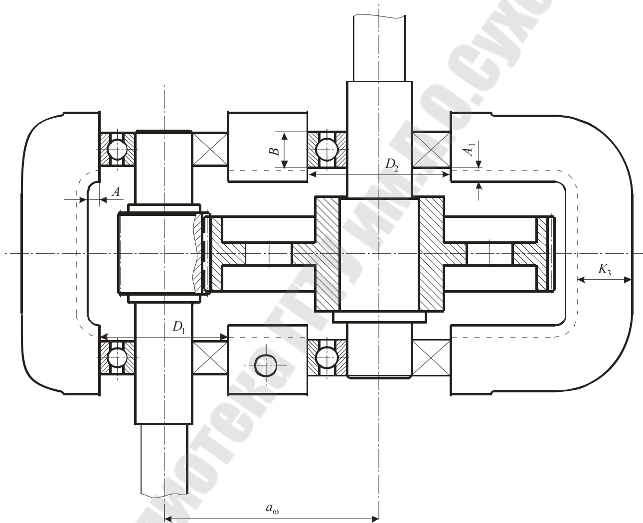
Рисунок 3 – Размещение подшипников
