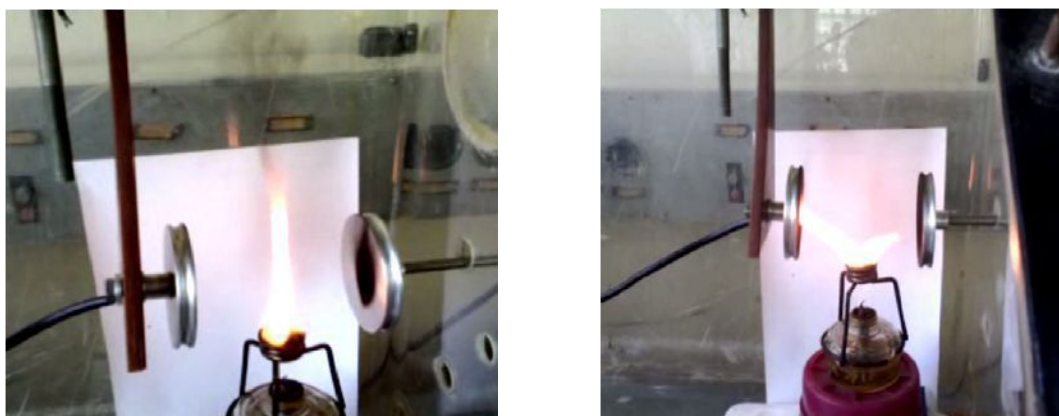
Рис. 4. Горение бензина в горизонтальном электрическом поле, отрицательный полюс слева: а – напряженность поля 20 кВ/м; б – напряженность поля 150 кВ/м
