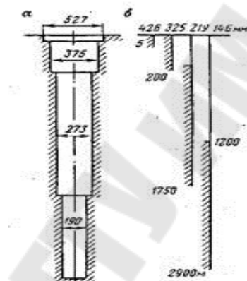
Рис. 2. Пример профиля (а) и рабочей схемы (в) конструкции скважины
