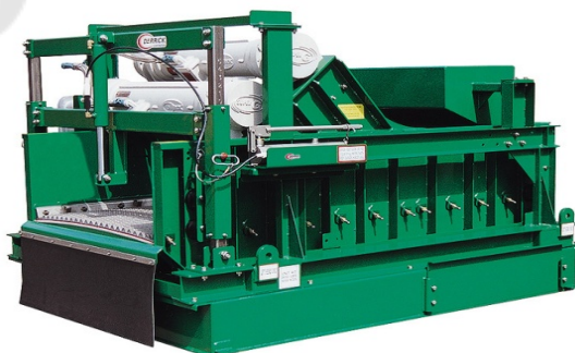
Рис. 6. Вибросито фирмы Derrick
