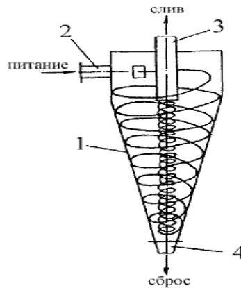
Рис. 7. Схема гидроциклона
