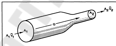
Рис.20. Непрерывность потока: скорость жидкости обратно пропорциональна площади поперечного сечения в направлении потока
