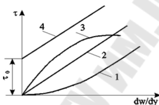
Рис.15. Реограммы жидкостей:
