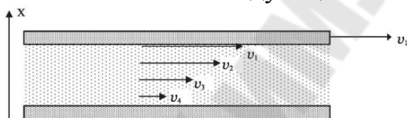
Рис.12. Течение вязкой жидкости между пластинами
