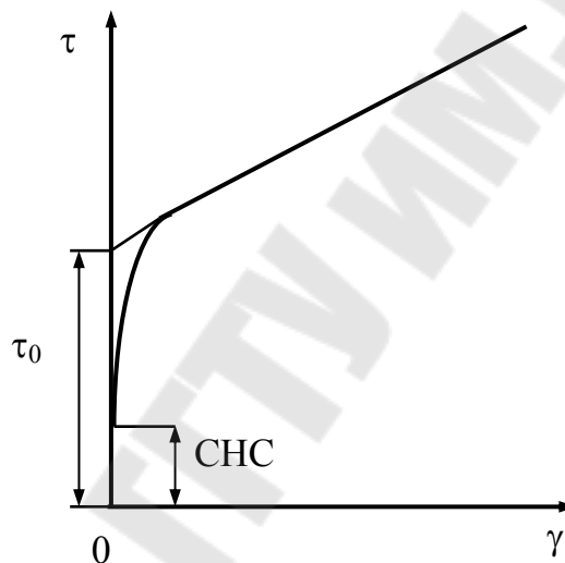
Рис. 16. Реограмма вязкопластичных жидкостей
