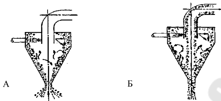
Рис.8. Разгрузка гидроциклона веером
