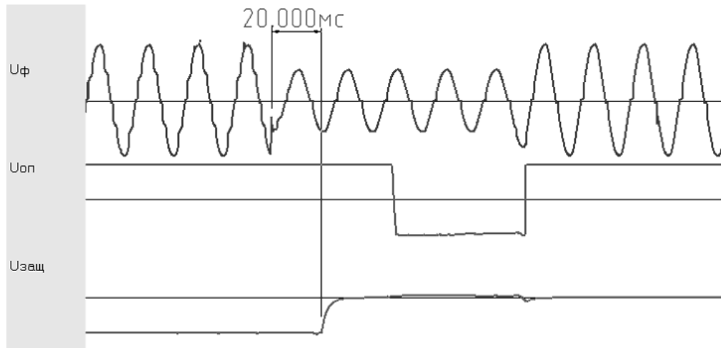
Рис. 1. Осциллограмма провала напряжения по цепи питания ( U_{\phi} ), опорного напряжения ( U_{оп} ) и напряжения узла защит ( U_{защ} ) тиристорного электропривода типа SSD
