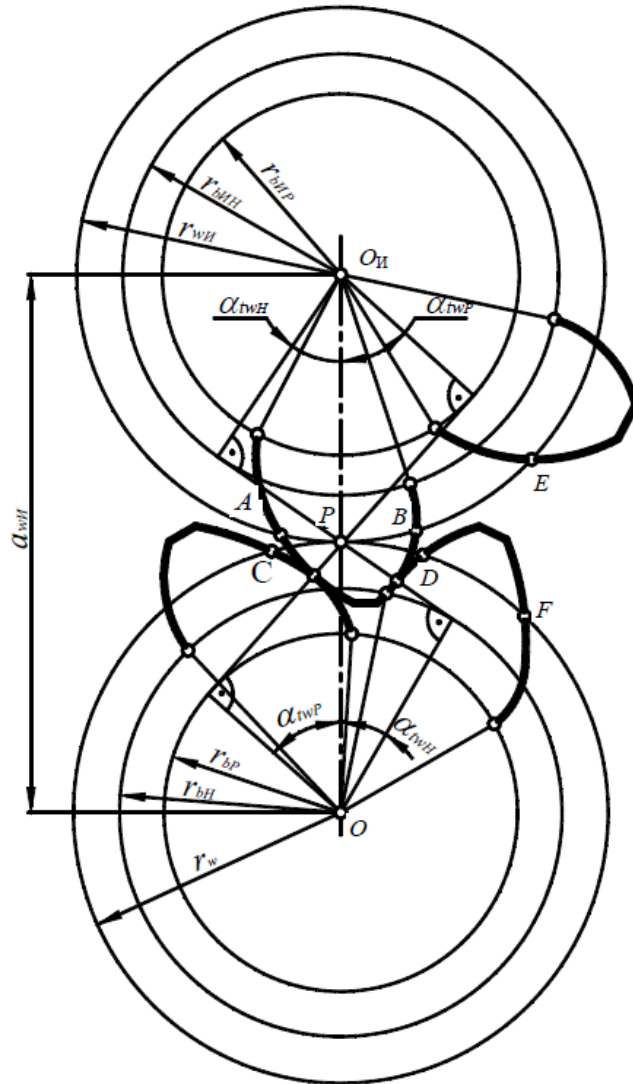
Рис. 2. Схема безззорного зацепления контролируемого и контрольного зубчатых колес в их торцовой плоскости: P – полюс зацепления
