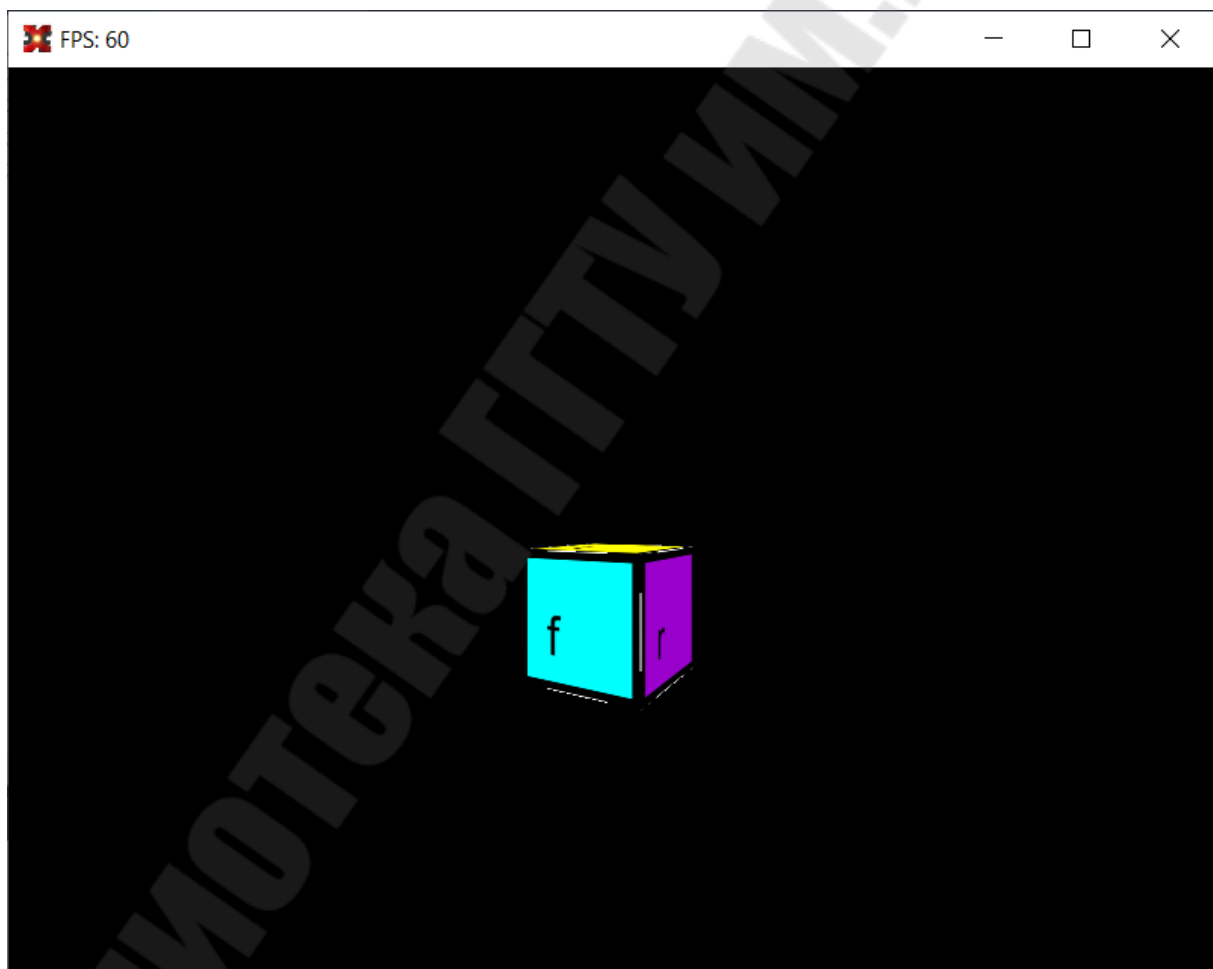
Рис. 3.4. Результат запуска
