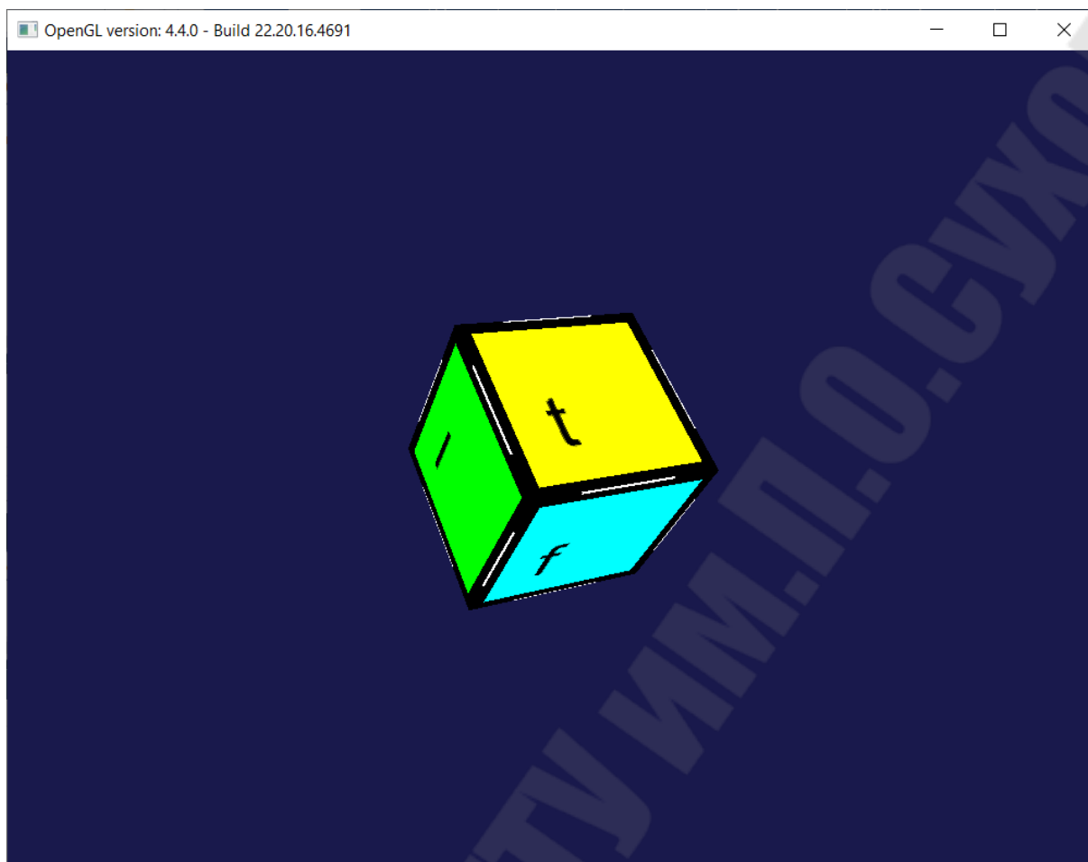
Рис. 5.3. Результат запуска
