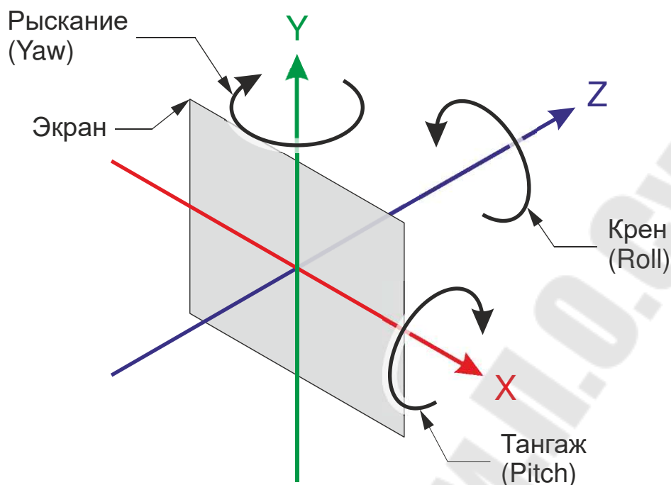
Рис. 2.4. Расположение осей относительно экрана в DirectX3D и углы поворота объектов в 3D пространстве
