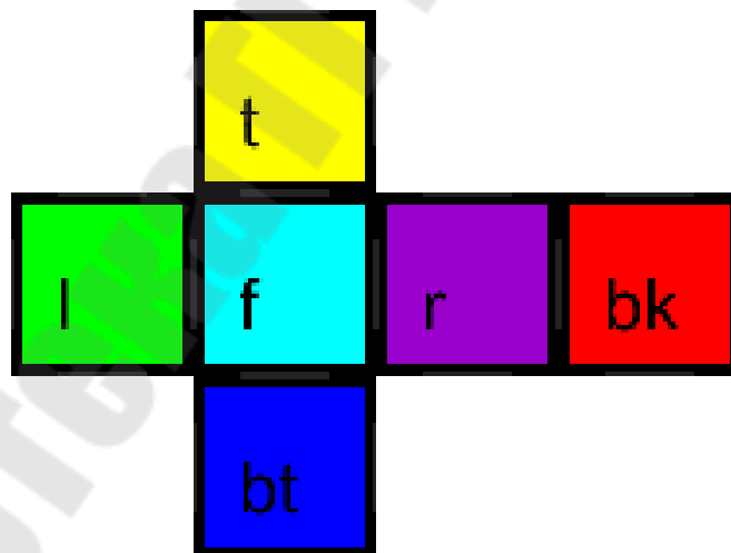
Рис. 5.2. Текстура куба
