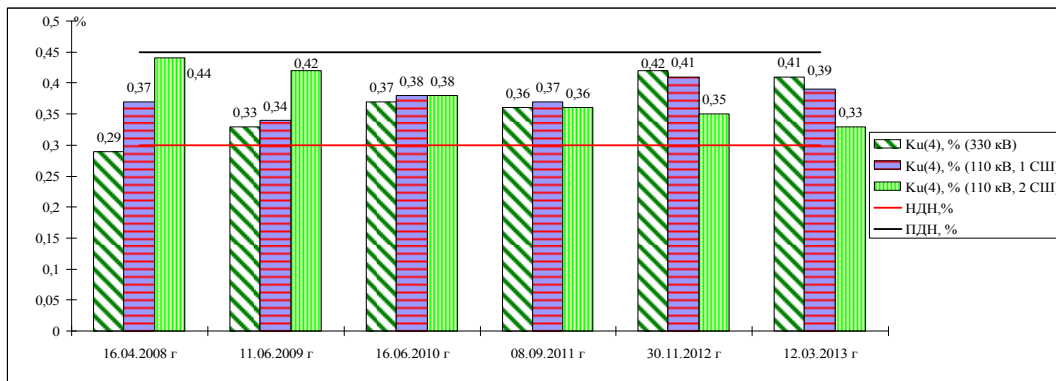
Рис. 4. График изменения коэффициента 4 гармонической составляющей напряжения K_{U(4)} на шинах 330 и 110 кВ подстанции «Прокат» РУП «БМЭ»
